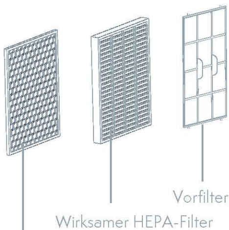
Aktivkohlefilter + Fotokatalysator
