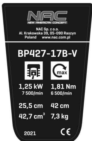
Tabliczka znamionowa
