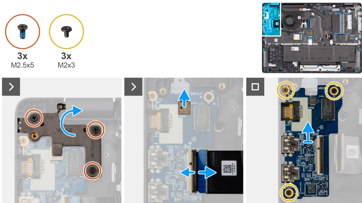
Rysunek 36. Wymontowywanie płyty we/wy
