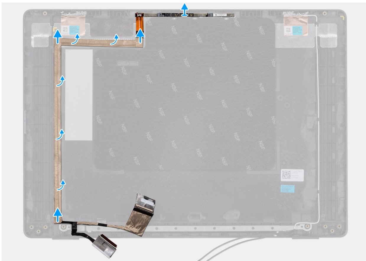
Rysunek 84. Wymontowywanie kabla eDP
