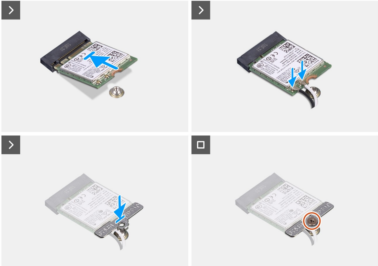
Rysunek 26. Instalowanie karty sieci bezprzewodowej
