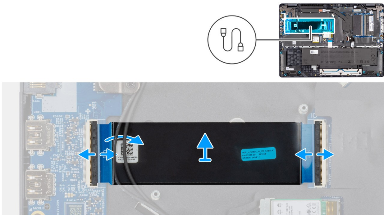
Rysunek 38. Wymontowywanie kabla FPC płyty we/wy
