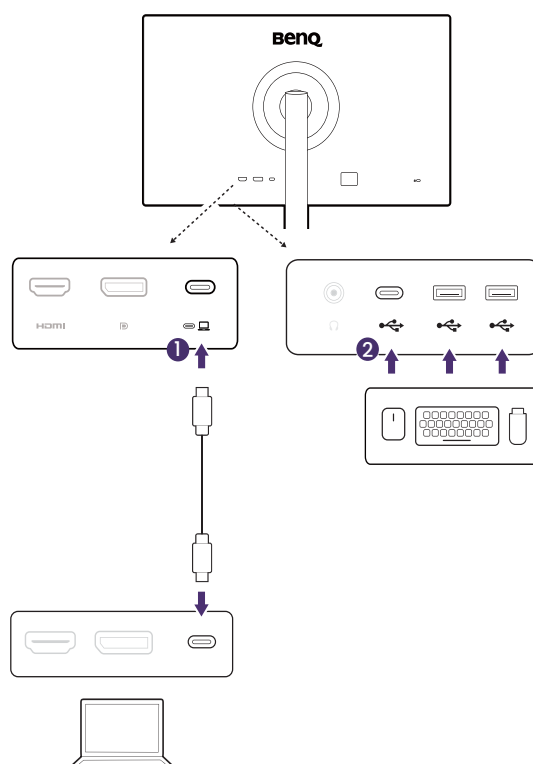
Wejście wideo przez USB-C™
