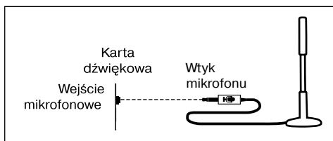
Rys. 1. Schemat połączeń
