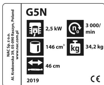
Tabliczka znamionowa
