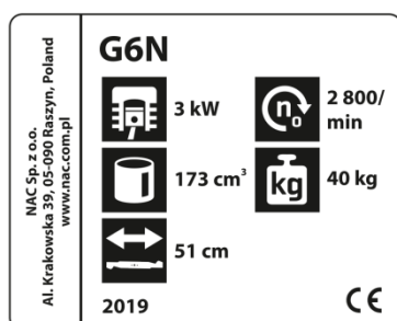
Tabliczka znamionowa
