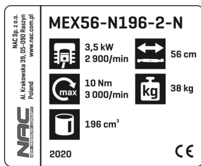
Tabliczka znamionowa
