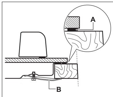
A) dołączona uszczelka
