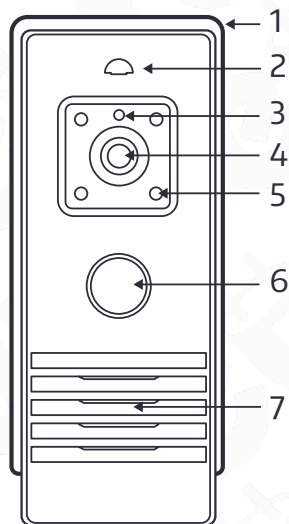
Rys. 2. Budowa kasety zewnętrznej
