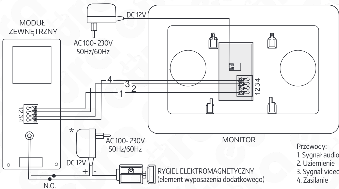
Rys. 6. Schemat połączeń zestawu
