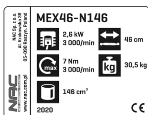
Tabliczka znamionowa
