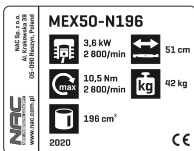
Tabliczka znamionowa
