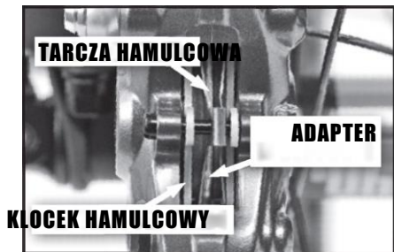
Sprawdzanie klocków hamulcowych w hamulcu Shimano – podkładka wspierająca nigdy nie powinna dotykać tarczy
