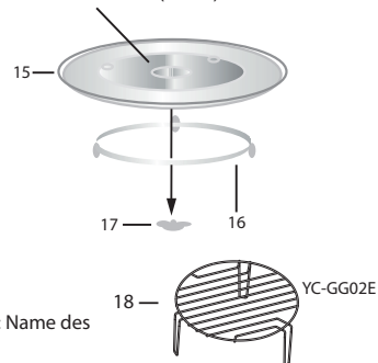
Drehkreuzeinlass (innen)
