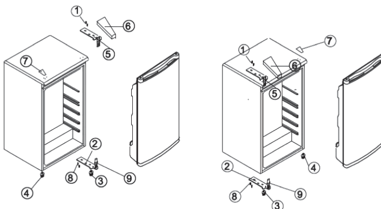
POŁOŻENIE ELEMENTÓW PRZED OBRÓCENIEM DRZWI
