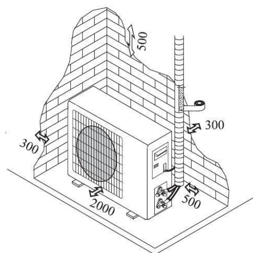
Minimalną wolną przestrzeń (mm) przedstawiono na rysunku:
