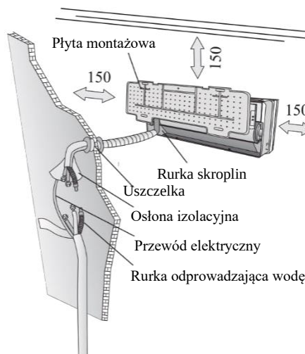
Minimalną wolną przestrzeń (mm) przedstawiono na rysunku:
