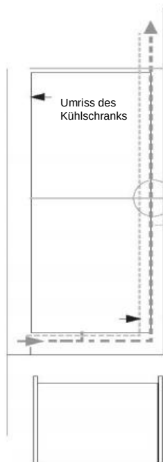
Draufsicht auf die Belüftungsöffnung auf der Rückseite
