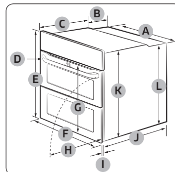
Piekarnik (mm)
