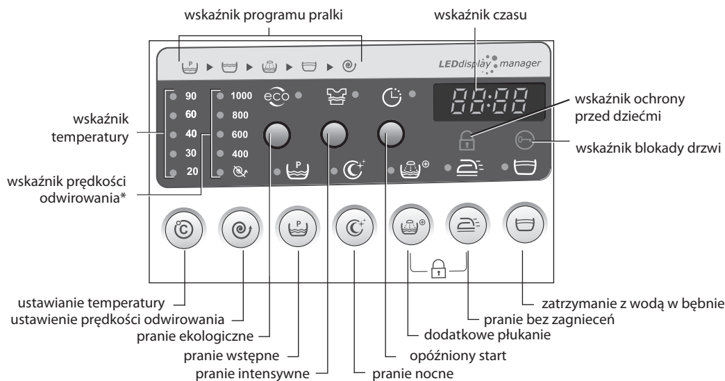
Rysunek 15 — Panel wskaźników i przycisków wyboru funkcji dodatkowych
