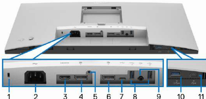
Widok od dołu monitora bez stojaka
