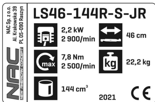
Tabliczka znamionowa
