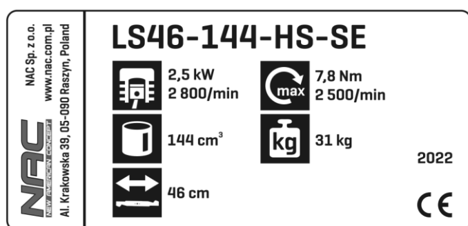
Tabliczka znamionowa
