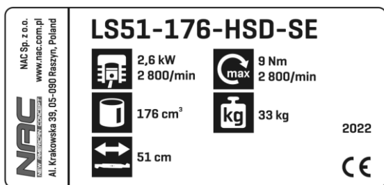
Tabliczka znamionowa
