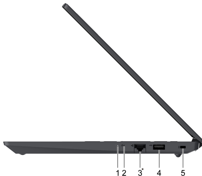
Rysunek 6. Widok z prawej strony—modele 14-calowe
