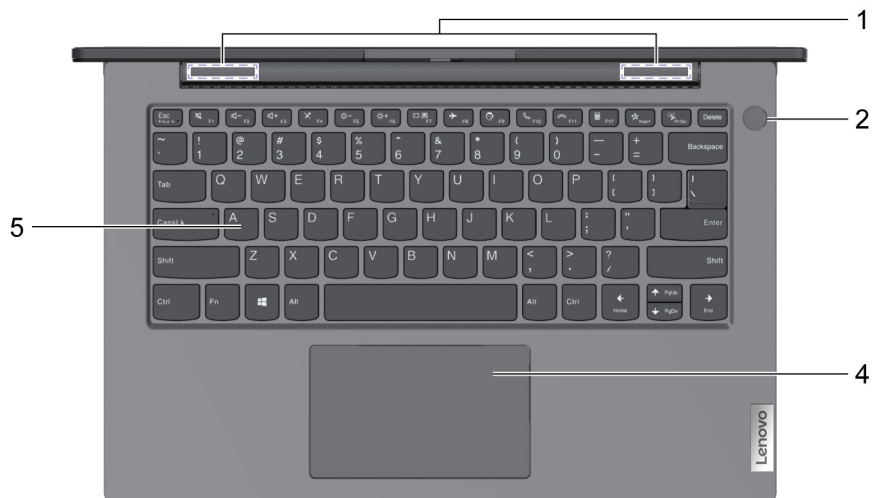
Rysunek 2. Widok podstawy—modele 14-calowe
