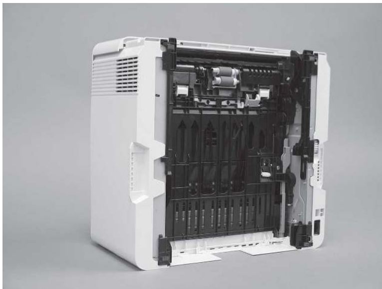
Rysunek 6-14 Umieść drukarkę spodem skierowanym do przodu
