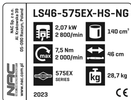
Tabliczka znamionowa
