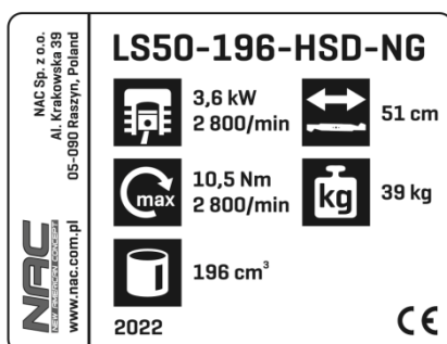
Tabliczka znamionowa
