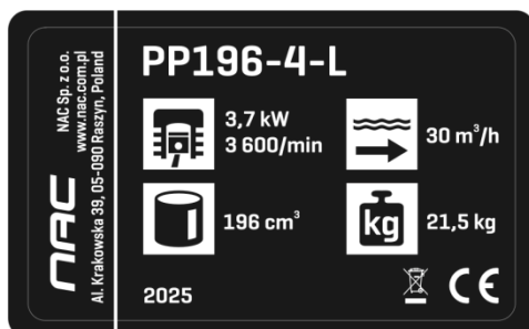
Tabliczka znamionowa
