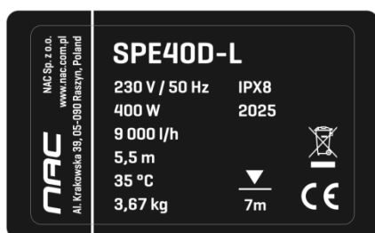
Przykładowa tabliczka znamionowa
