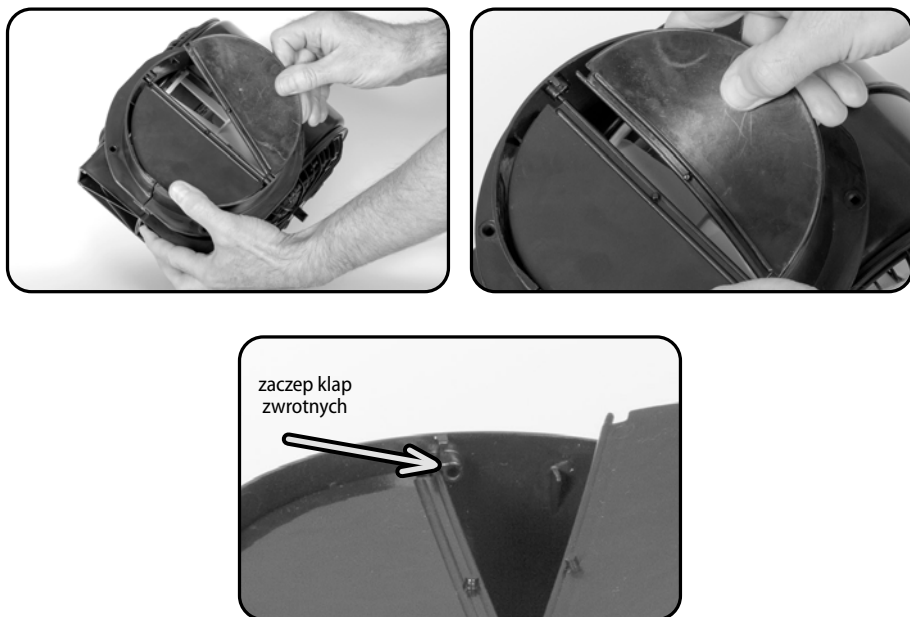
Ryc. 4. Montaż klapy zwrotnej na wylocie turbiny
