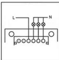
Odetnij zasilanie, podłącz przewody i dokręć śruby.
