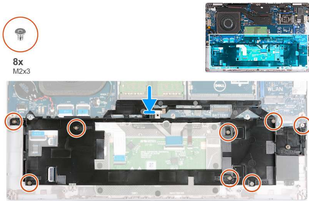
Rysunek 34. Instalowanie zestawu ramy montażowej
