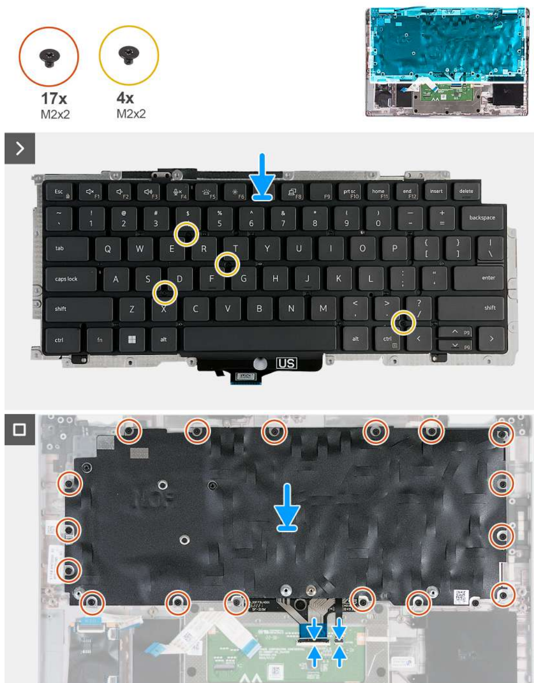
Rysunek 66. Instalowanie klawiatury
