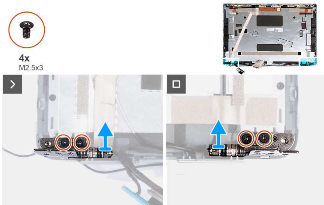
Rysunek 49. Wymontowywanie zawiasów wyświetlacza
