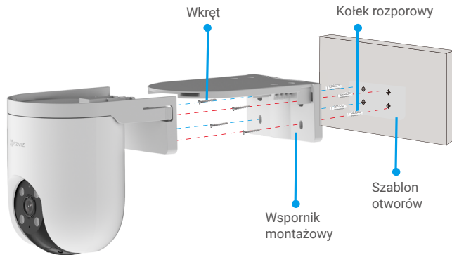
Rys. 2 Montaż ścienny
