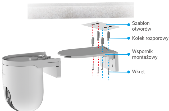
Rys. 1 Montaż sufitowy
