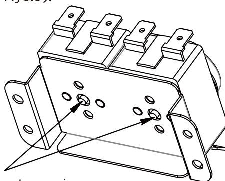
Przycisk resetowania ręcznego
