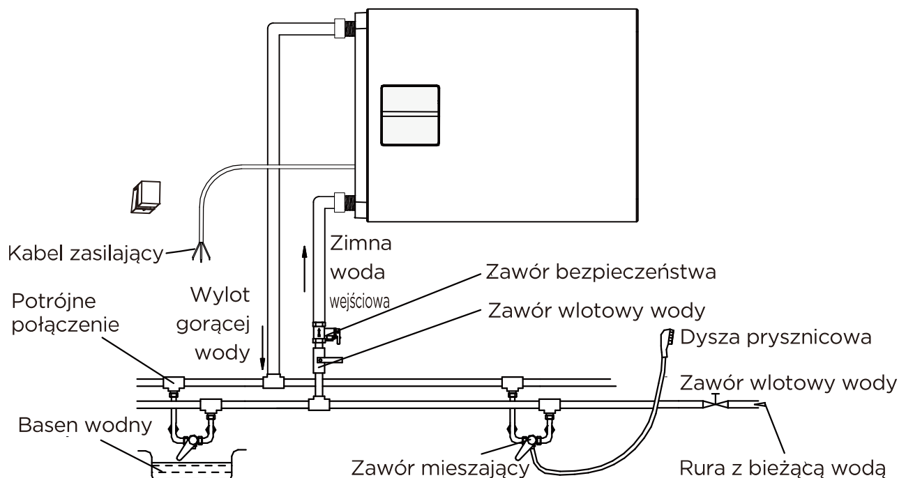
↑ INSTALACJA POZIOMA
