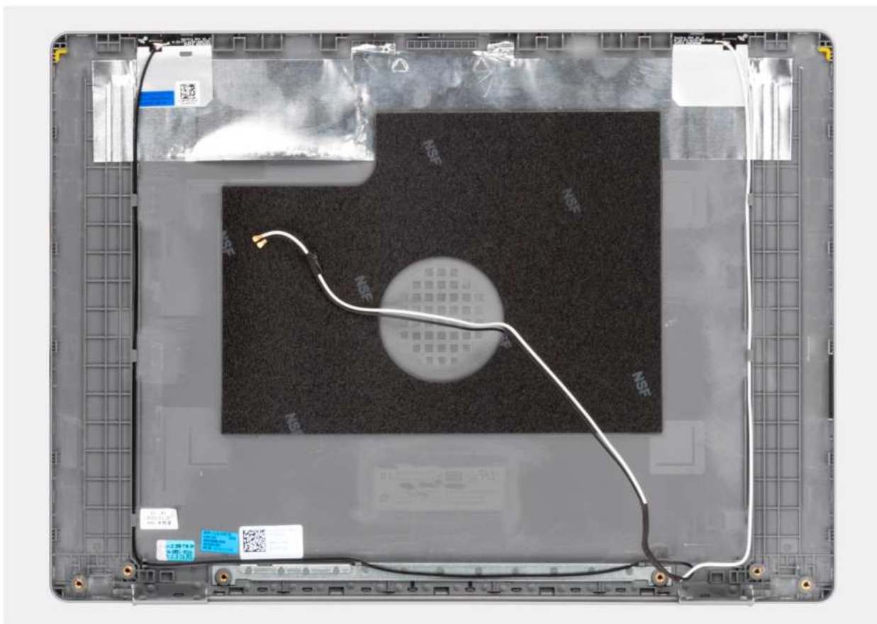
Rysunek 66. Zestaw pokrywy wyświetlacza i anteny
