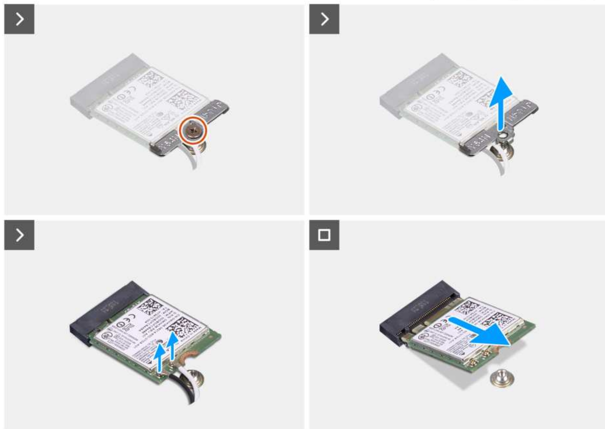
Rysunek 18. Wymontowywanie karty sieci bezprzewodowej
