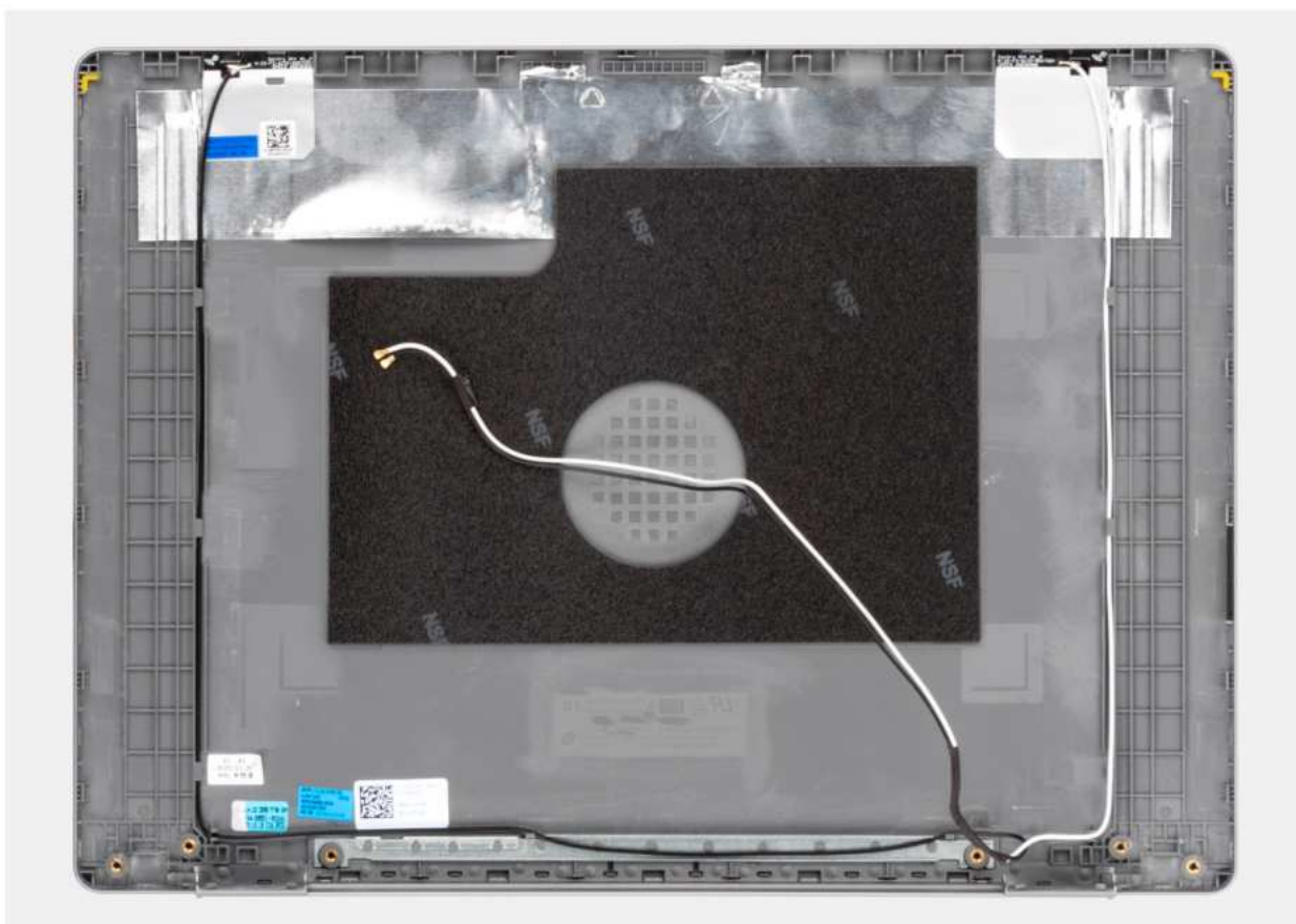
Rysunek 67. Zestaw pokrywy wyświetlacza i anteny
