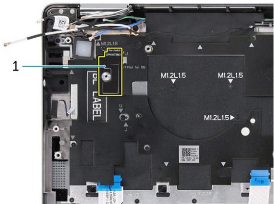
Rysunek 64. Płyta nośna klawiatury komputera w konfiguracji z kartą sieci WWAN 4G
