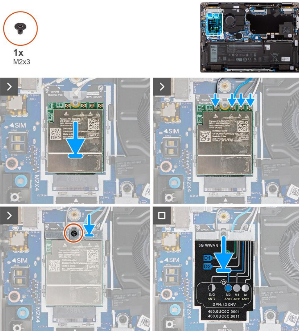
Rysunek 24. Instalowanie karty sieci WWAN
