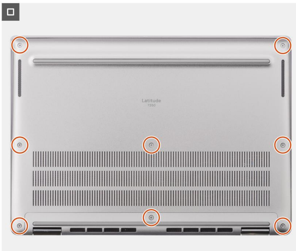
Rysunek 20. Instalowanie pokryw dolnej
