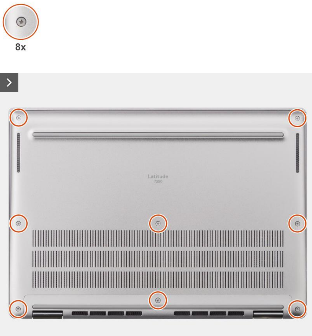
Rysunek 15. Wymontowywanie pokrywy dolnej
