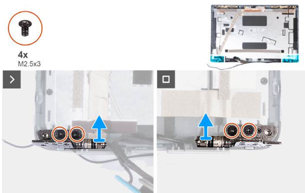
Rysunek 60. Wymontowywanie zawiasów wyświetlacza
