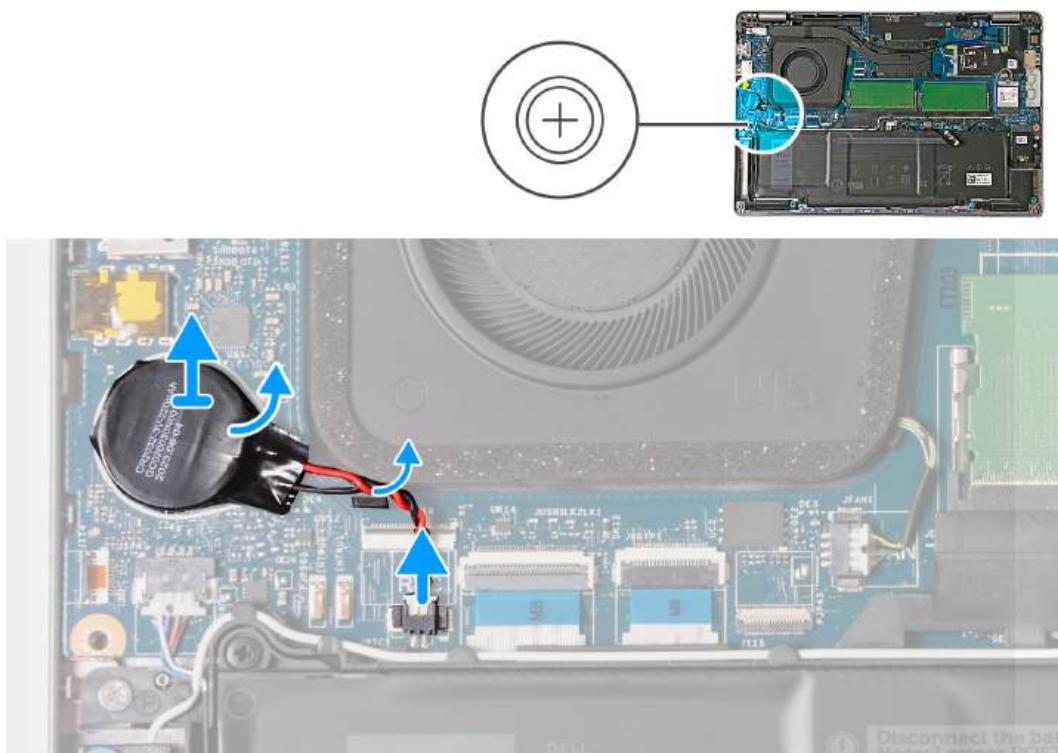
Rysunek 28. Wymontowywanie baterii pastylkowej
