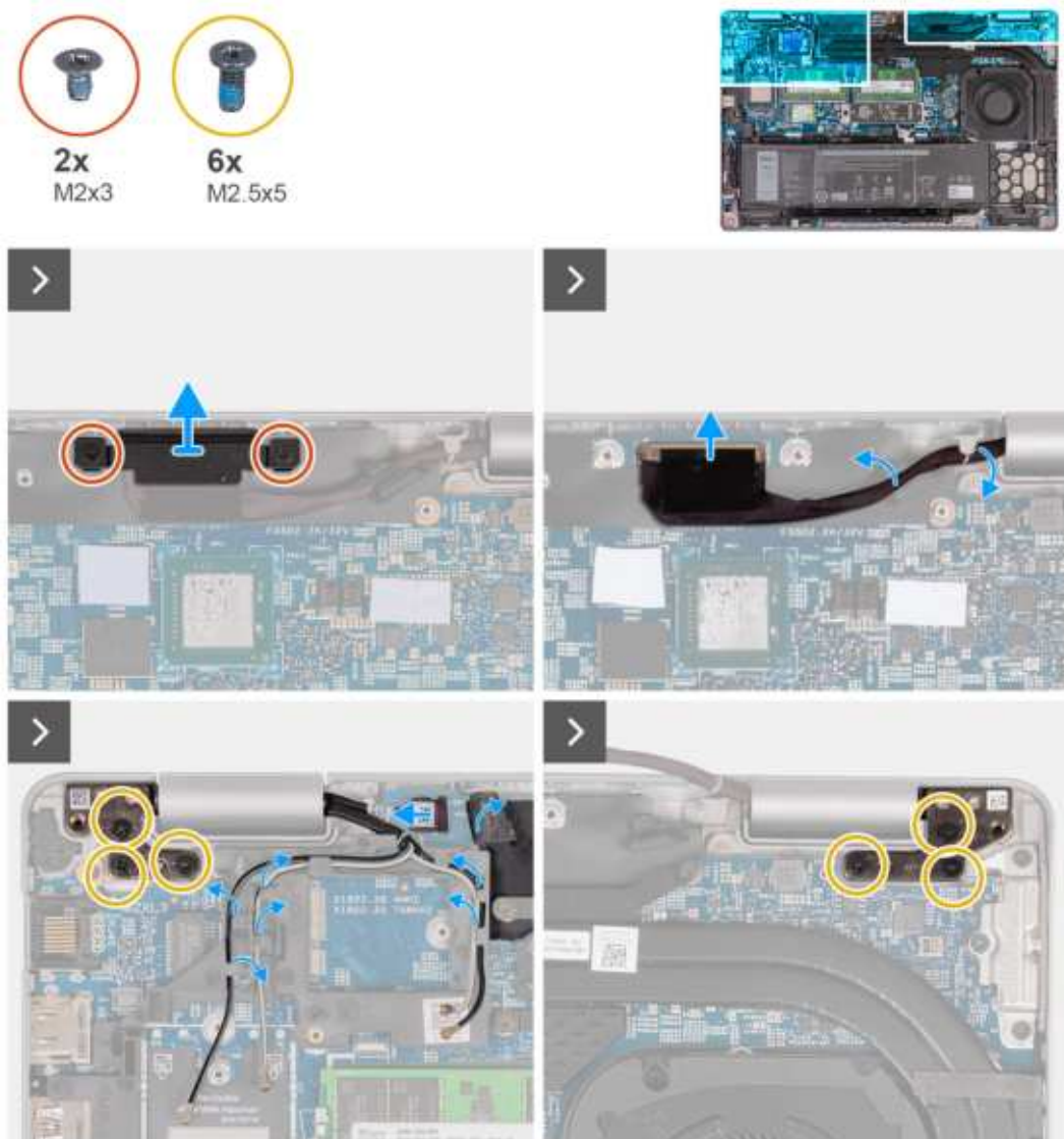
Rysunek 69. Wymontowywanie zestawu wyświetlacza
