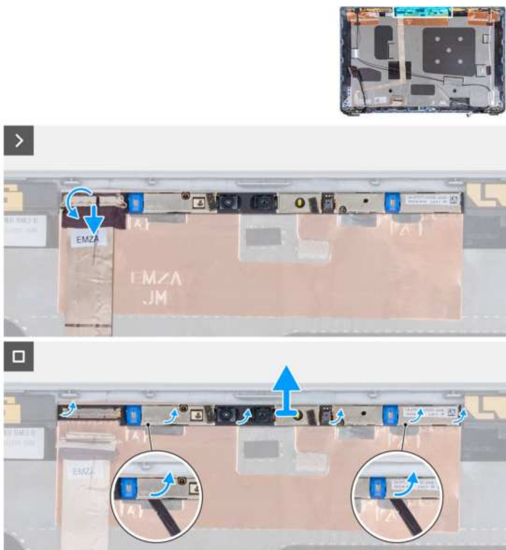
Rysunek 84. Wymontowywanie modułu kamery
