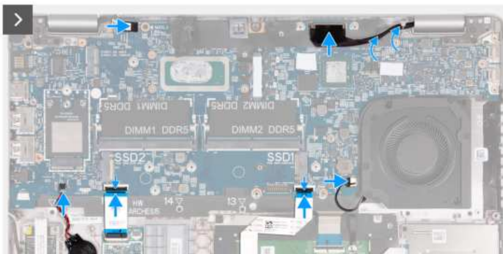
Rysunek 59. Instalowanie płyty głównej
