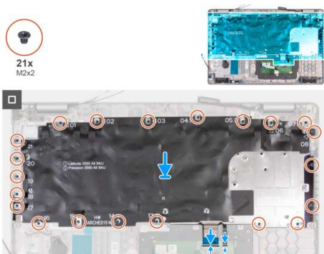
Rysunek 68. Instalowanie klawiatury
