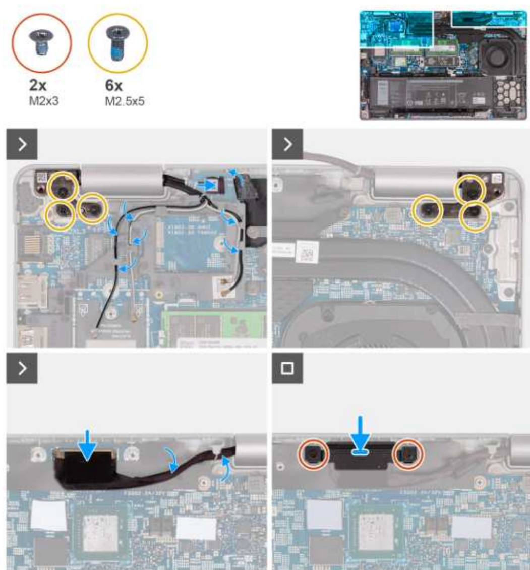
Rysunek 73. Instalowanie zestawu wyświetlacza
