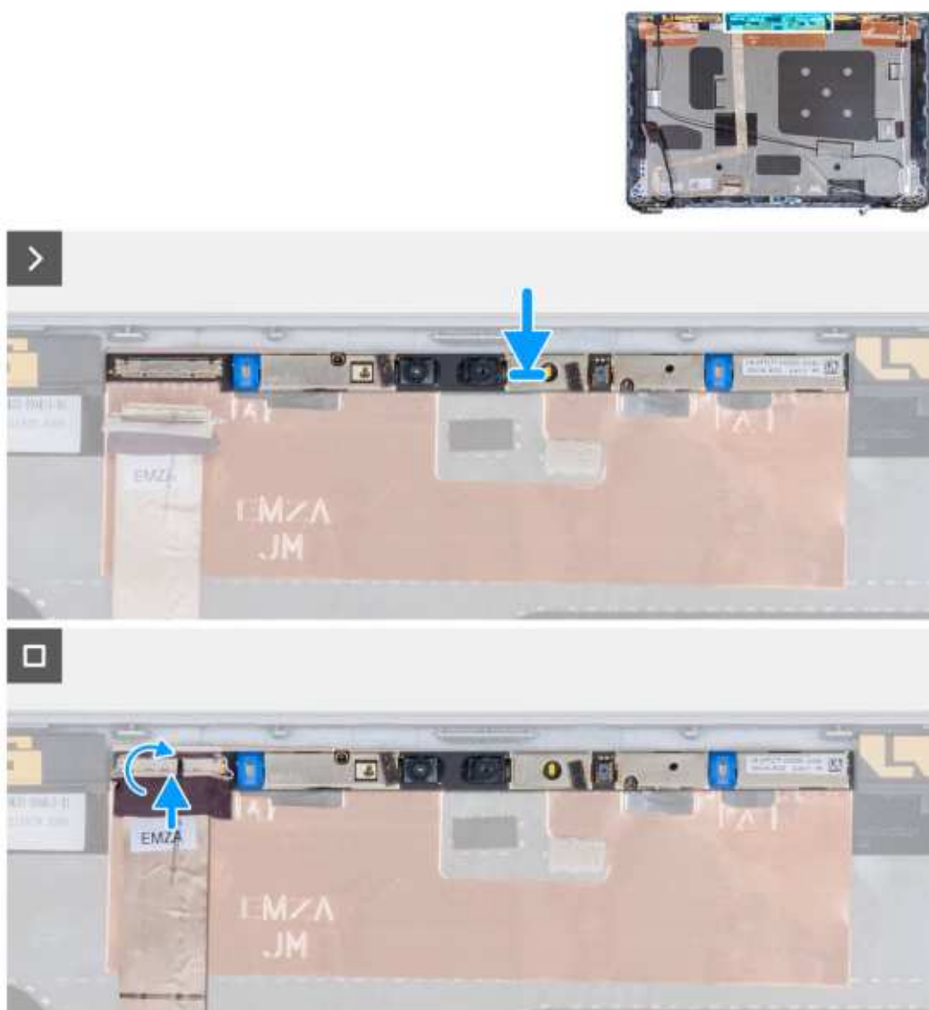
Rysunek 85. Instalowanie modułu kamery
