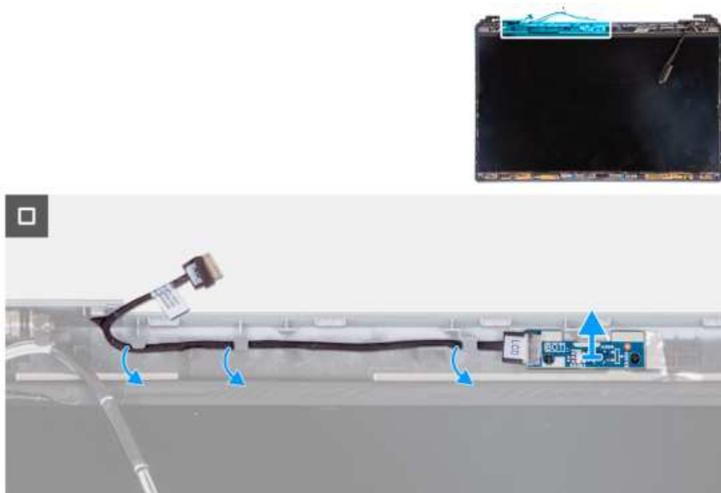
Rysunek 92. Wymontowywanie płyty czujników
