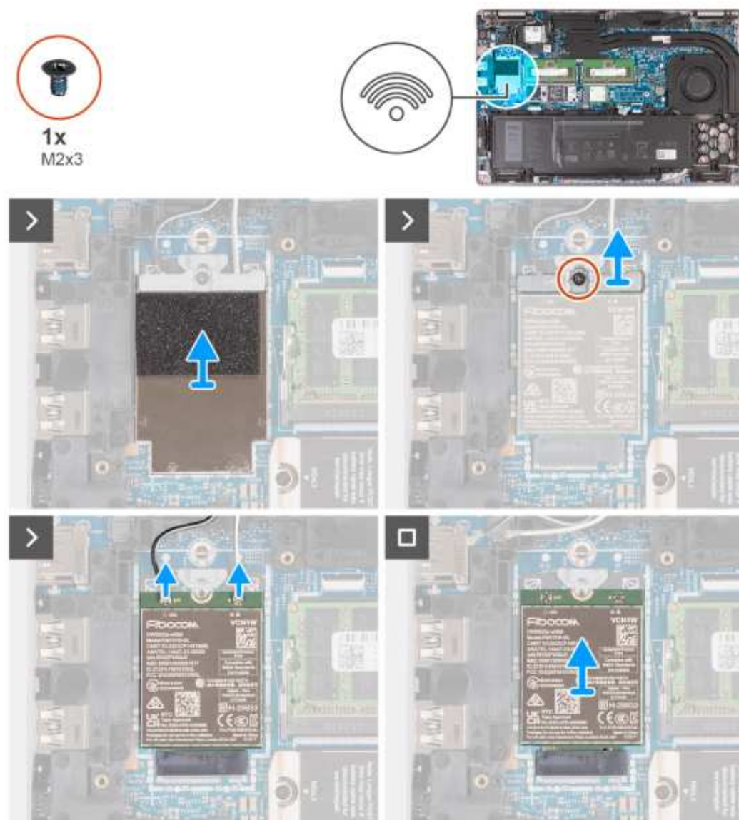
Rysunek 21. Wymontowywanie karty sieci WWAN 4G
