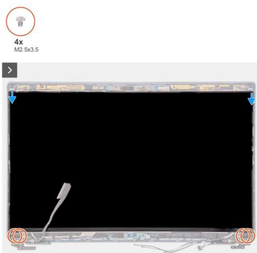
Rysunek 76. Wymontowywanie wyświetlacza
