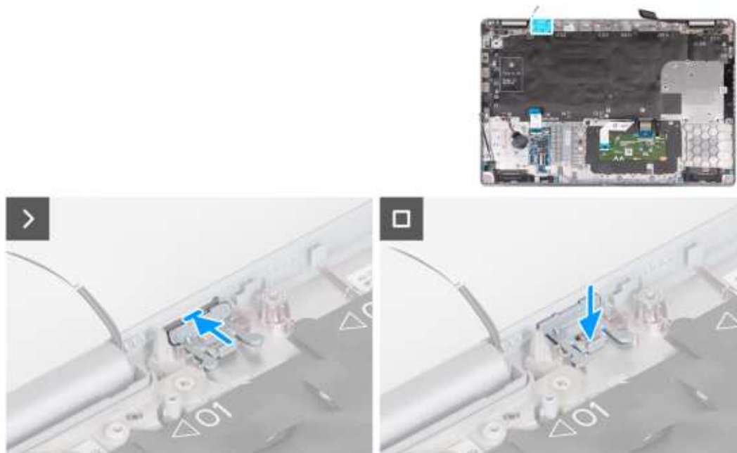
Rysunek 99. Instalowanie zaślepki gniazda karty SIM
