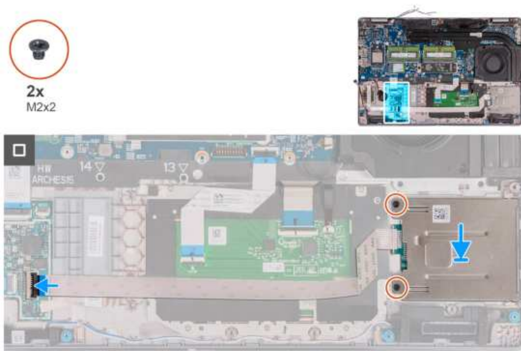
Rysunek 97. Instalowanie czytnika kart smart
