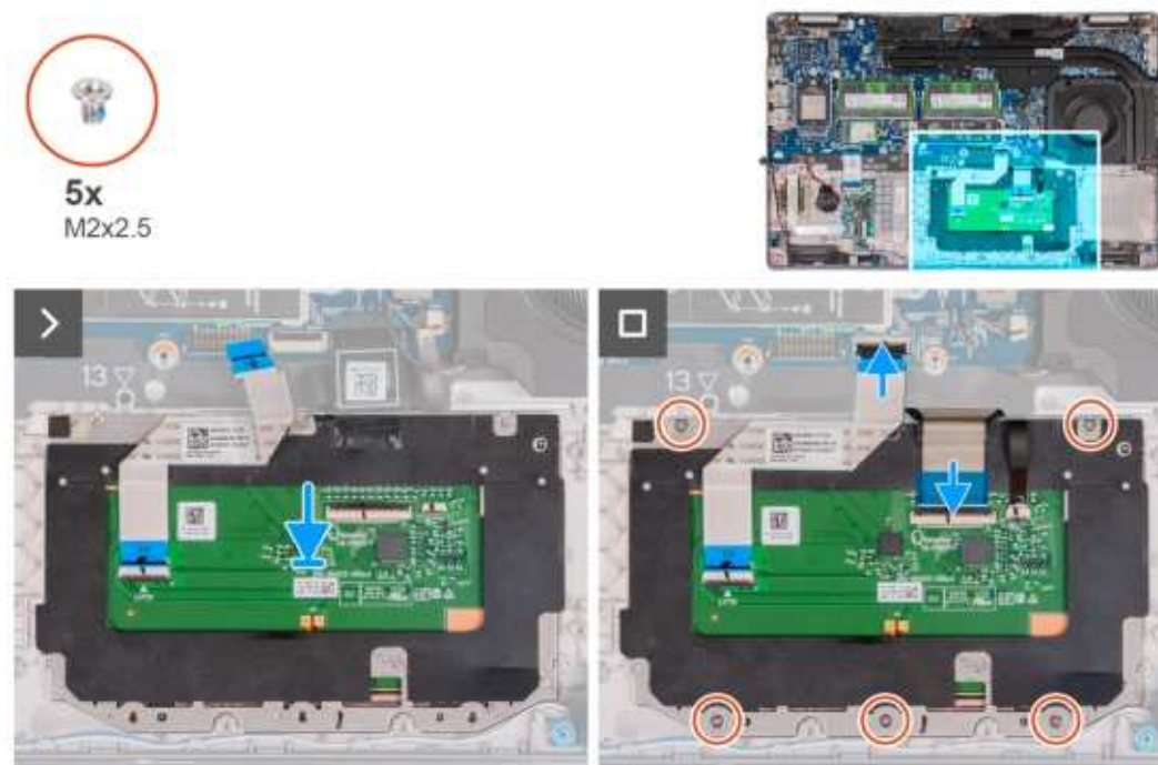
Rysunek 42. Instalowanie touchpada
