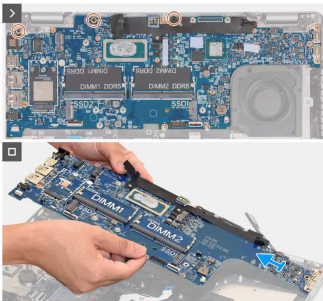
Rysunek 55. Wymontowywanie płyty głównej
