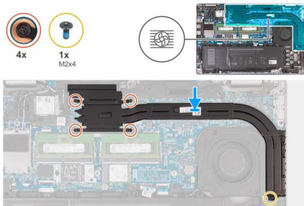
Rysunek 51. Instalowanie radiatora (zintegrowana karta graficzna)
