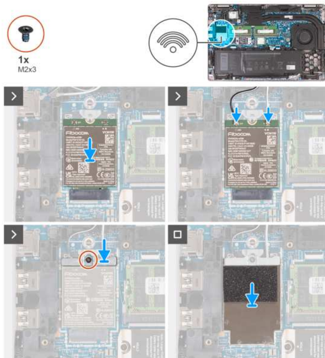
Rysunek 22. Instalowanie karty sieci WWAN 4G
