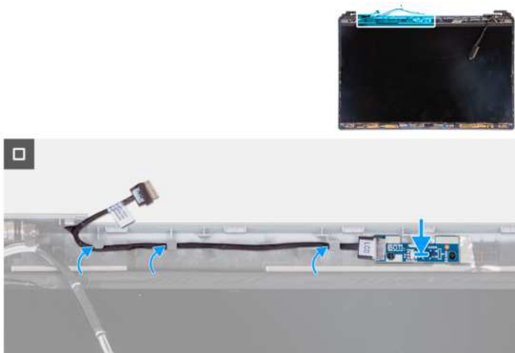
Rysunek 93. Instalowanie płyty czujników
