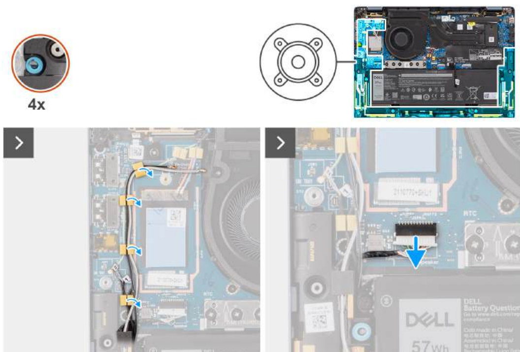
Rysunek 26. Wymontowywanie głośników — dotyczy komputerów w konfiguracji Ultralight
