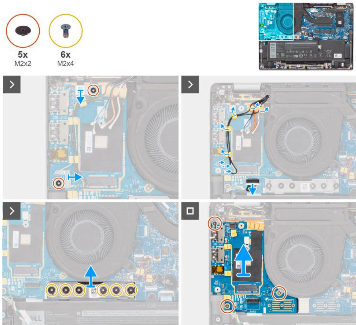
Rysunek 68. Wymontowywanie karty towarzyszącej we/wy
