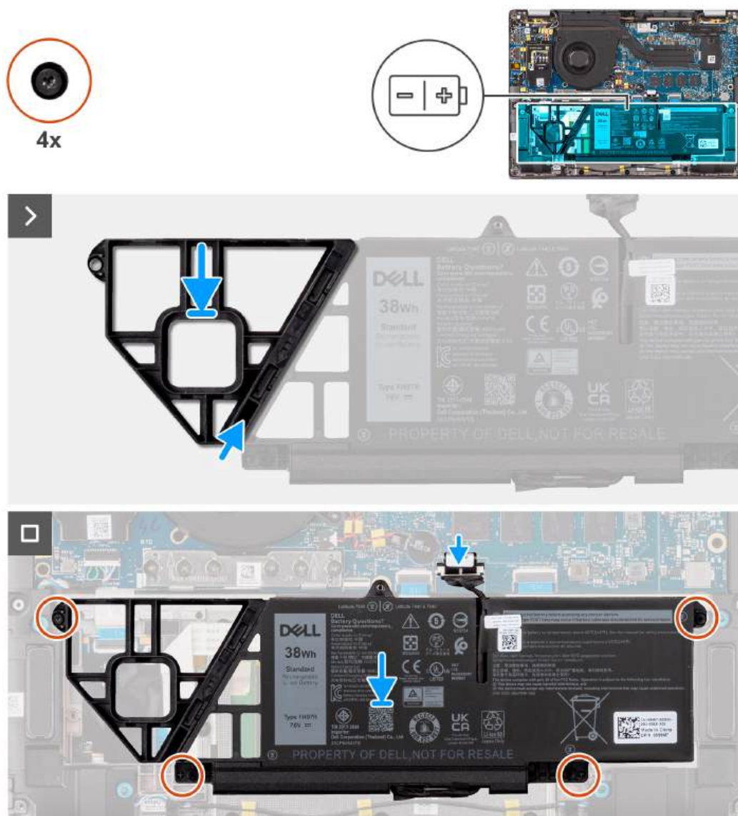
Rysunek 36. Instalowanie baterii 2-ogniowej
