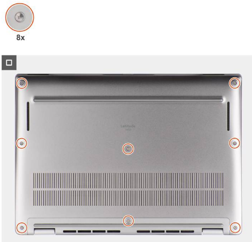
Rysunek 18. Instalowanie pokrywy dolnej
