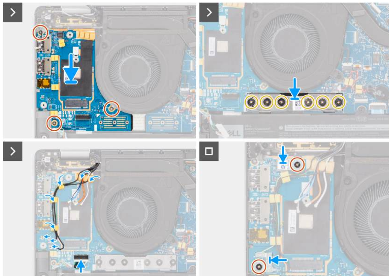
Rysunek 72. Instalowanie karty towarzyszącej we/wy
