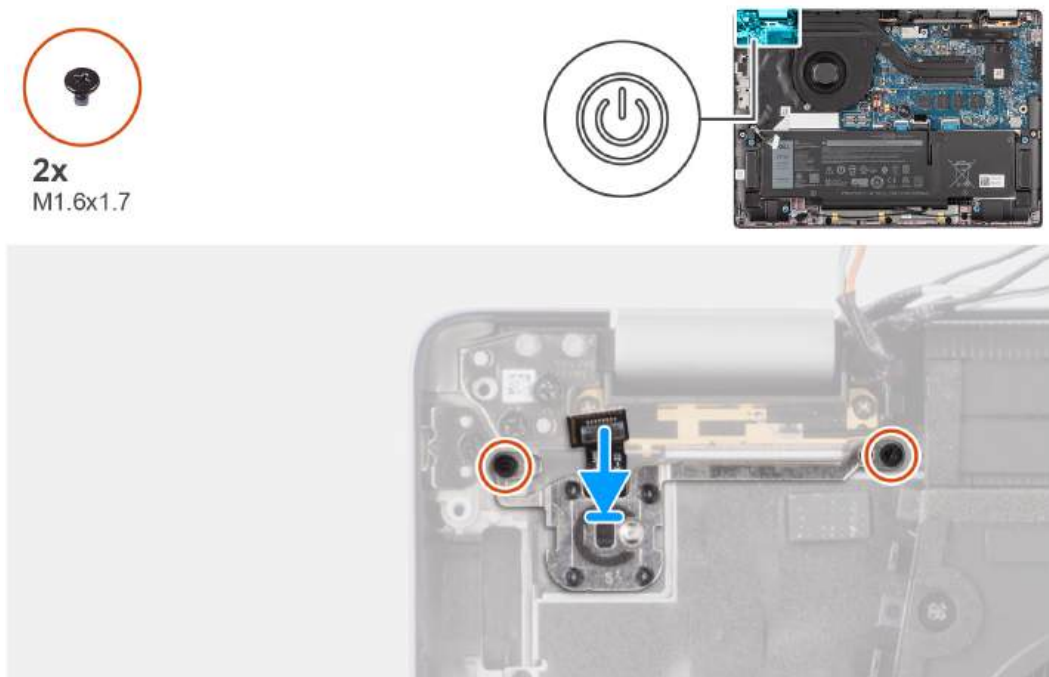
Rysunek 74. Instalowanie przycisku zasilania z opcjonalnym czytnikiem linii papilarnych
