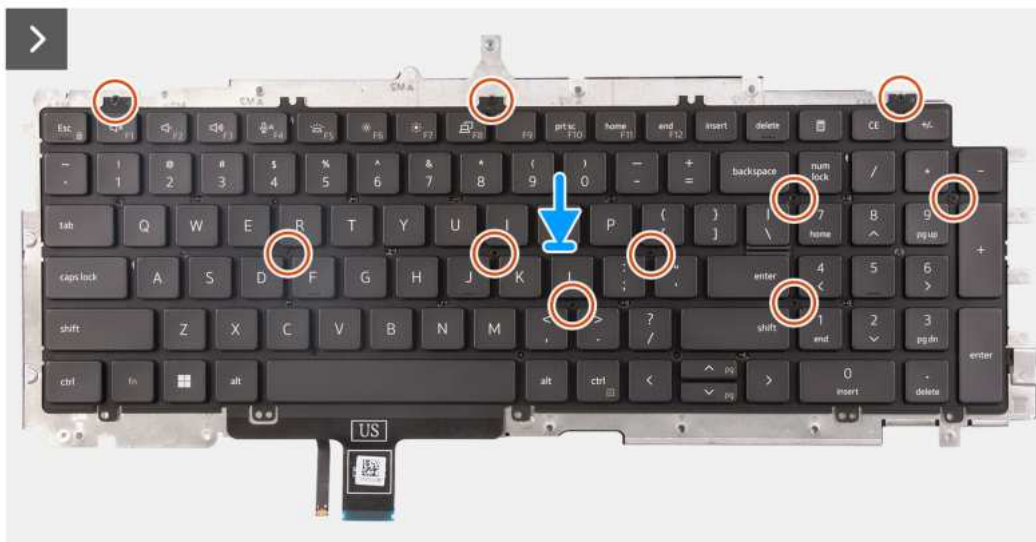
Rysunek 67. Instalowanie klawiatury
