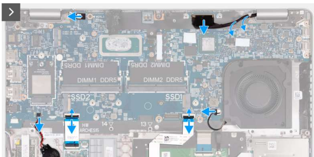
Rysunek 54. Ilustracja: odłączanie kabli płyty głównej
