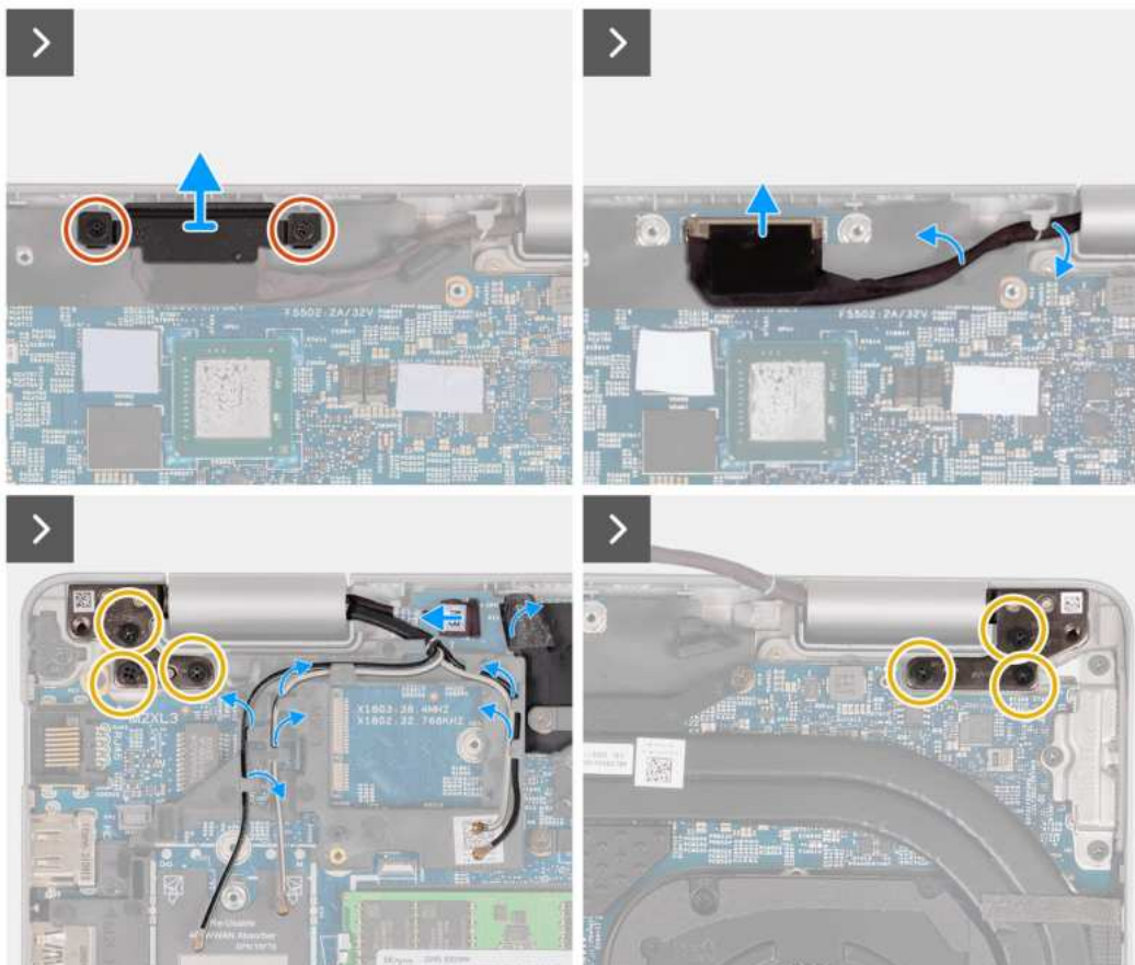
Rysunek 69. Wymontowywanie zestawu wyświetlacza
