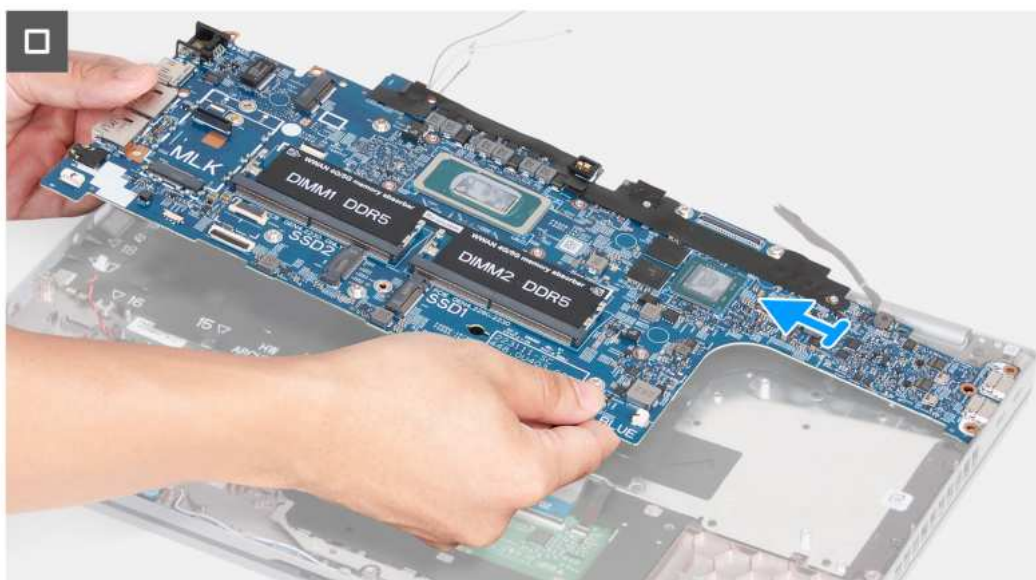
Rysunek 56. Wymontowywanie płyty głównej
