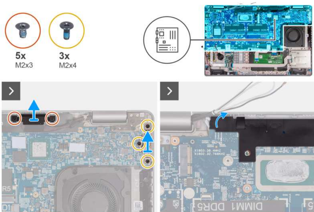
Rysunek 53. Wykręcanie śrub
