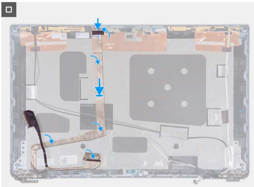
Rysunek 91. Instalowanie kabla wyświetlacza
