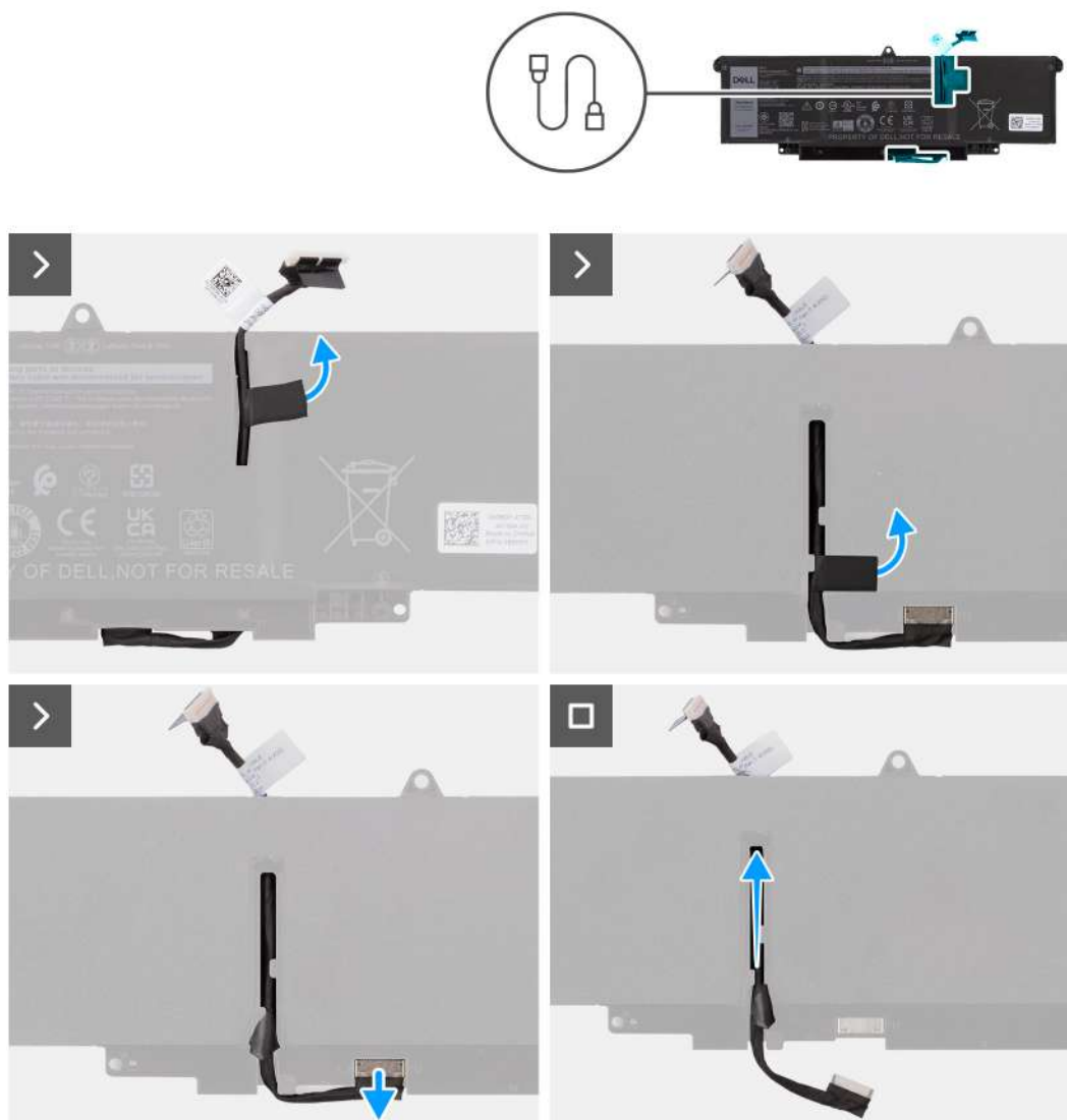
Rysunek 31. Wymontowywanie kabla baterii
