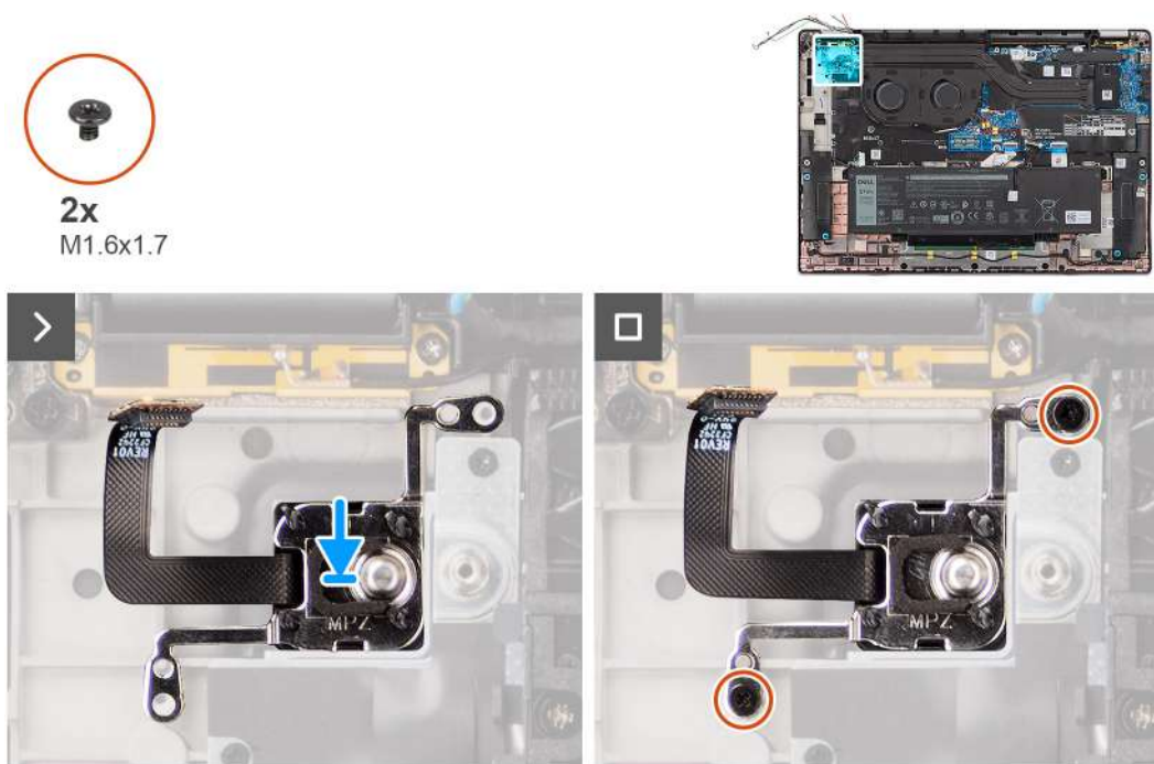
Rysunek 63. Instalowanie przycisku zasilania z opcjonalnym czytnikiem linii papilarnych
