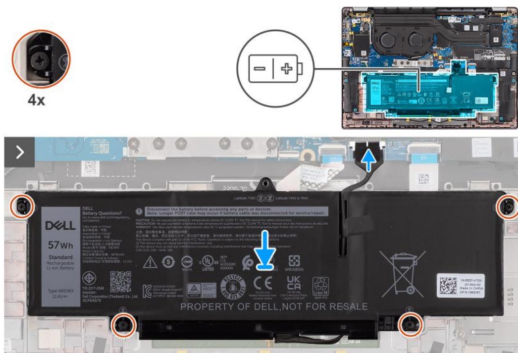
Rysunek 30. Instalowanie baterii 3-ogniowej
