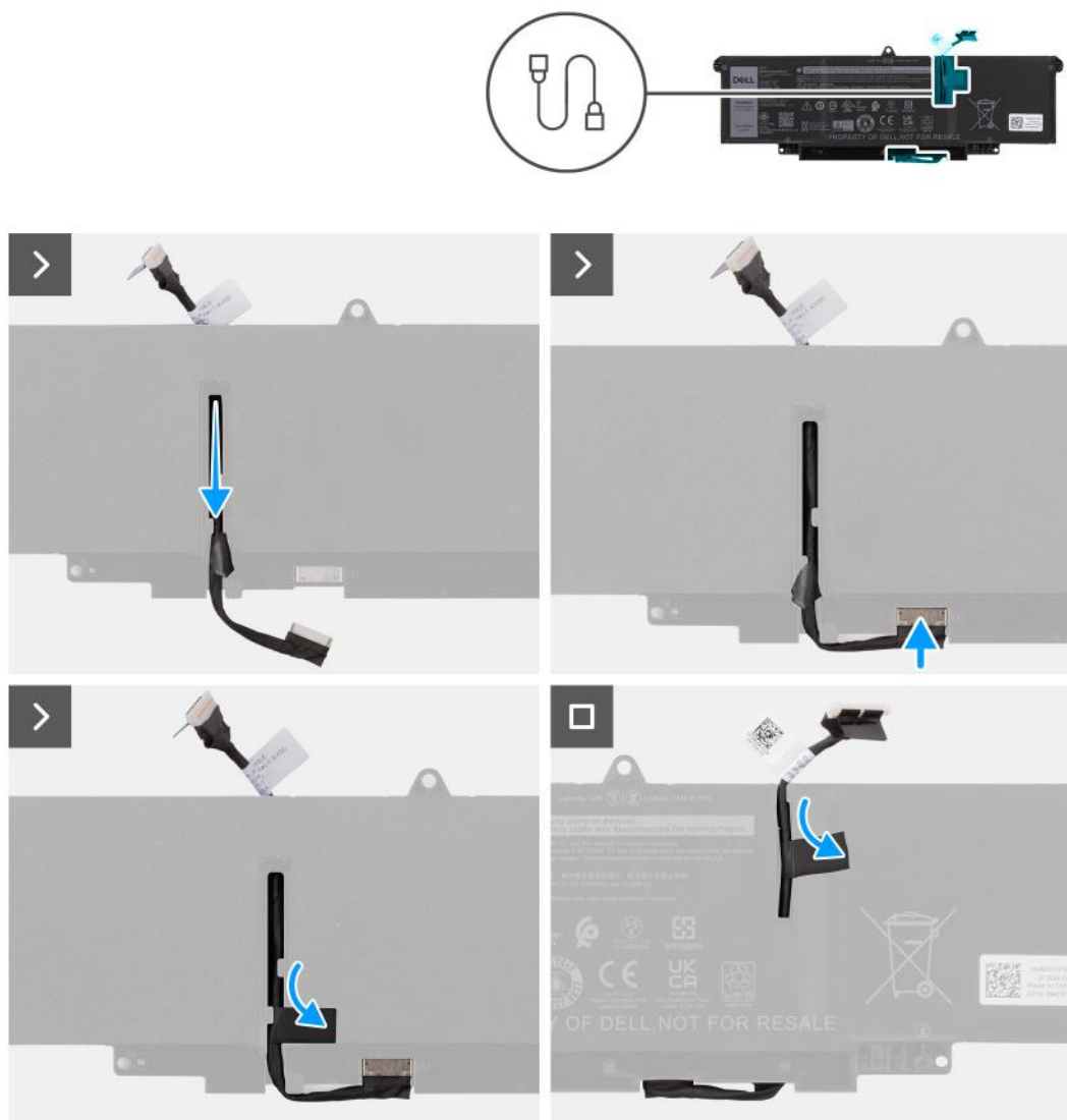
Rysunek 32. Instalowanie kabla baterii
