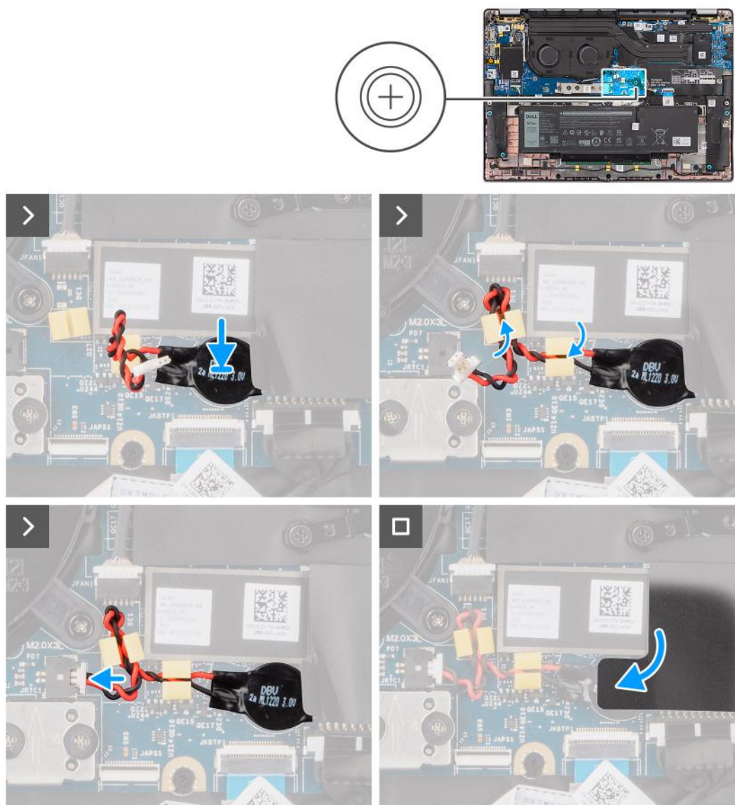
Rysunek 25. Instalowanie baterii pastylkowej
