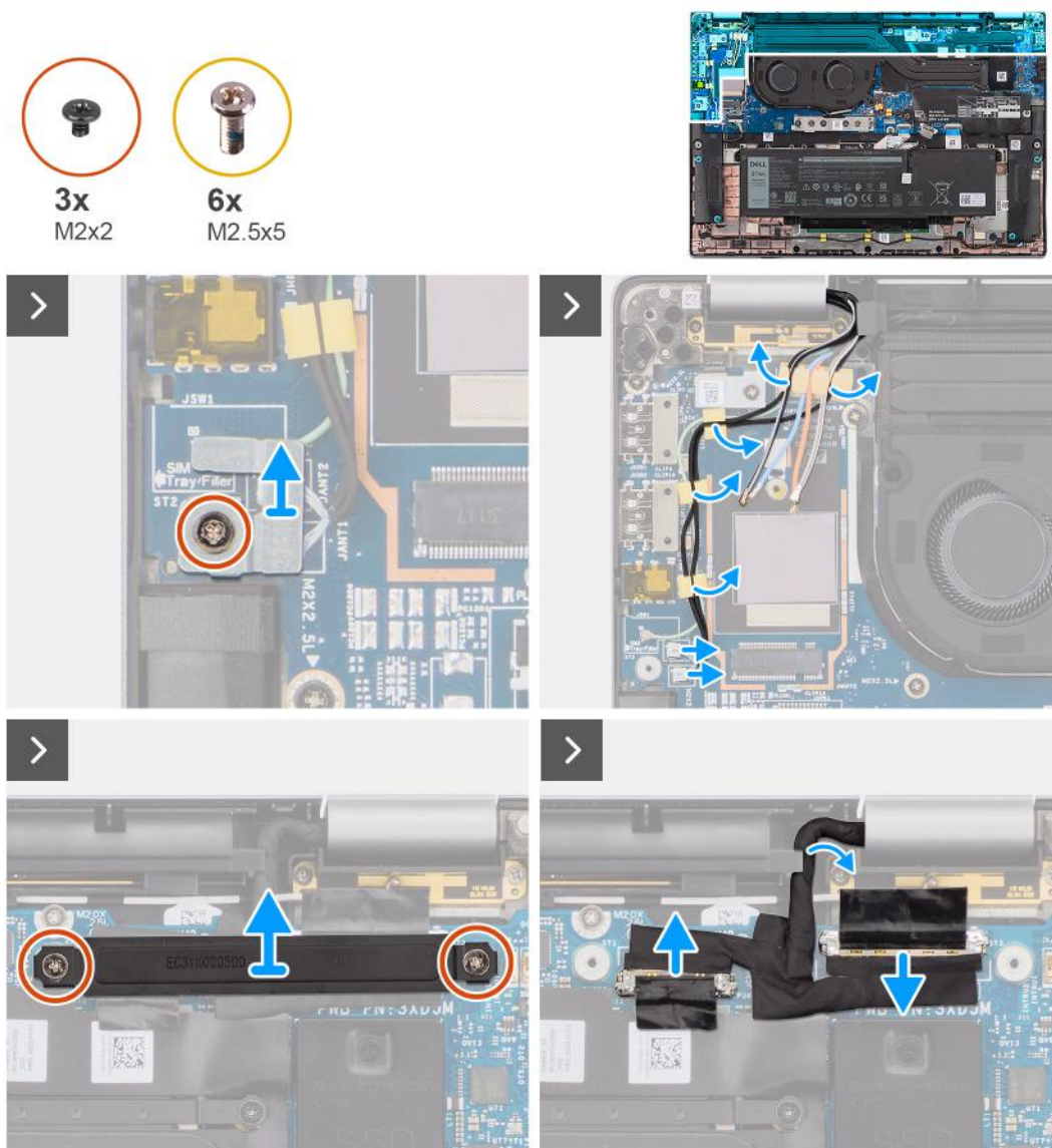
Rysunek 35. Wymontowywanie zestawu wyświetlacza
