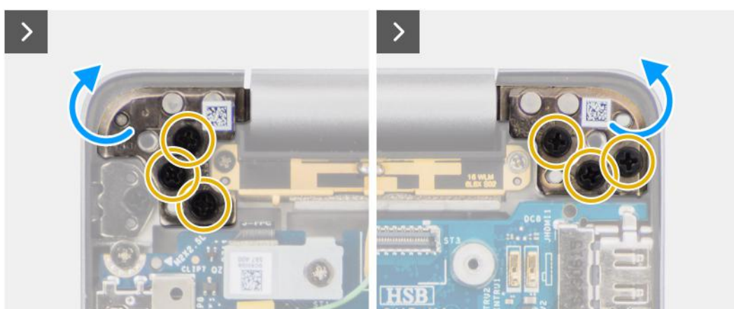
Rysunek 36. Wymontowywanie zestawu wyświetlacza
