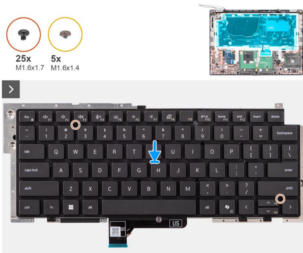
Rysunek 66. Instalowanie klawiatury
