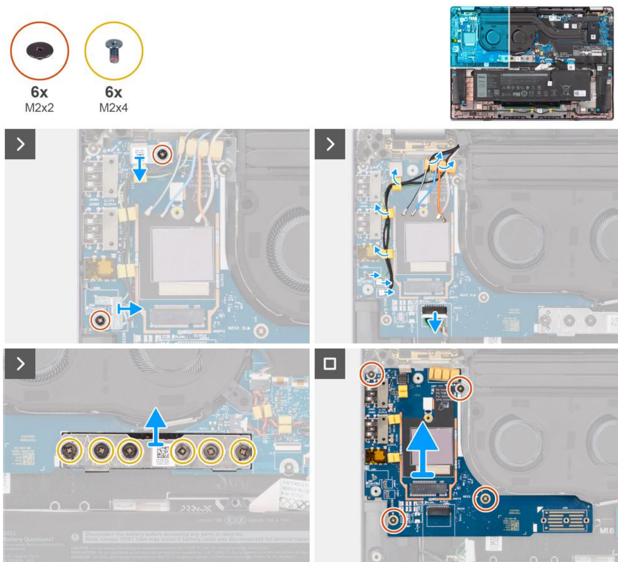
Rysunek 58. Wymontowywanie karty towarzyszącej we/wy
