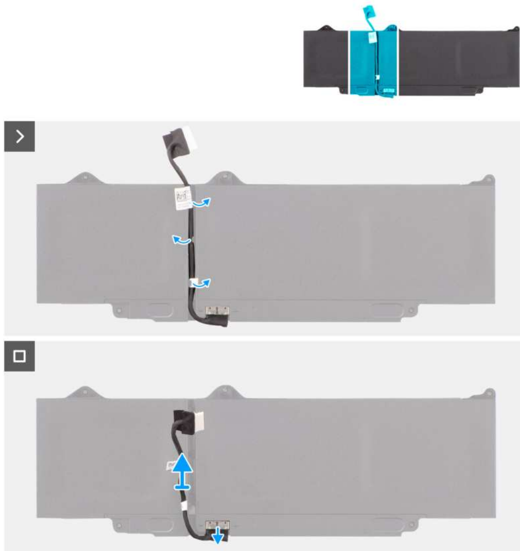
Rysunek 25. Wymontowywanie kabla baterii
