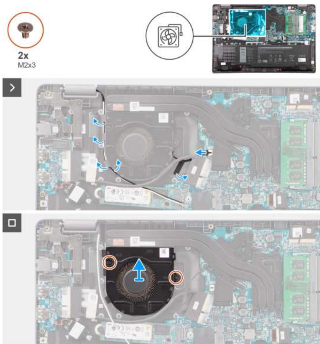
Rysunek 33. Wymontowywanie wentylatora
