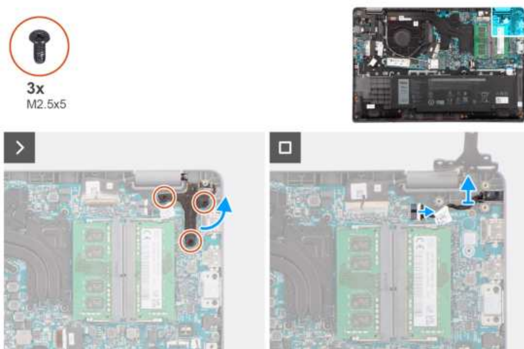
Rysunek 27. Wymontowywanie gniazda zasilacza
