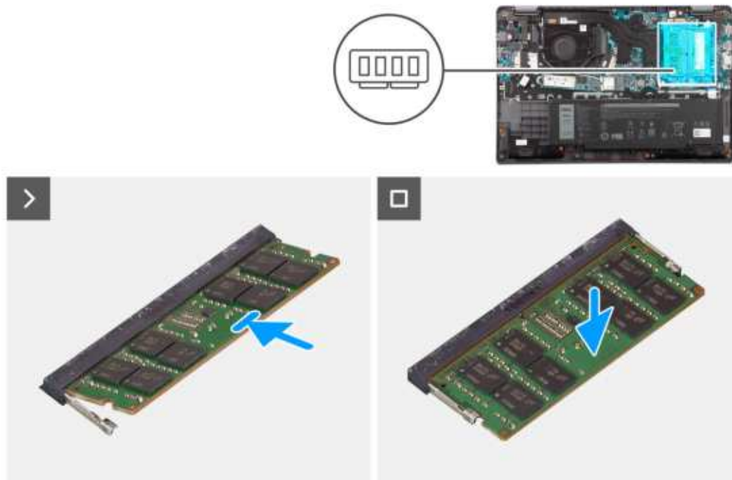
Rysunek 13. Instalowanie modułów pamięci
