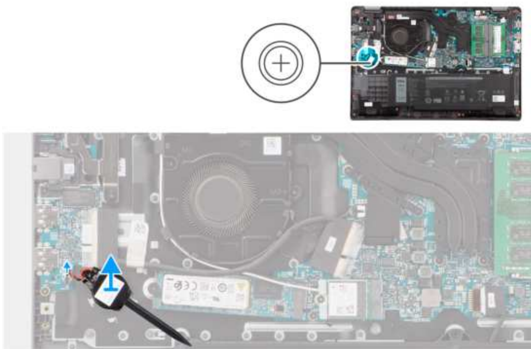
Rysunek 18. Wymontowywanie baterii pastylkowej
