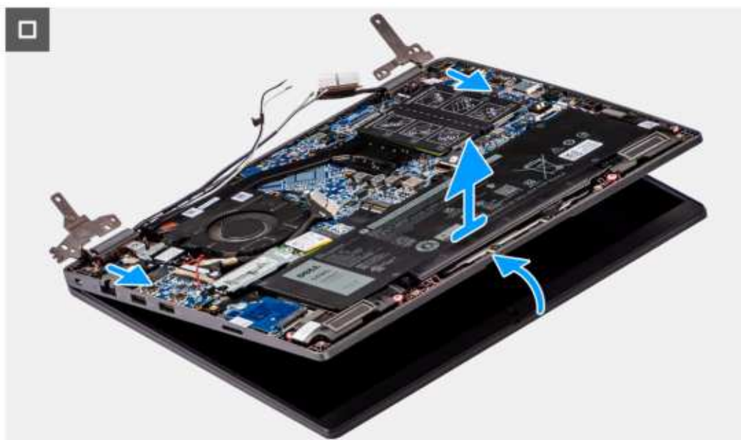
Rysunek 49. Wymontowywanie zestawu wyświetlacza
