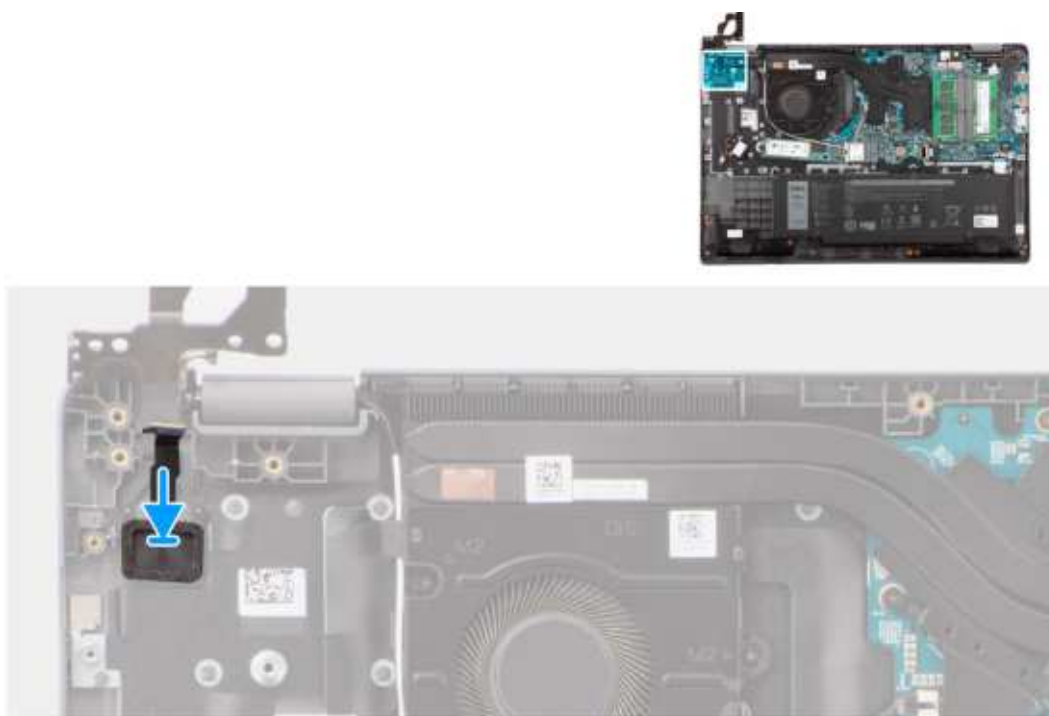
Rysunek 40. Instalowanie przycisku zasilania
