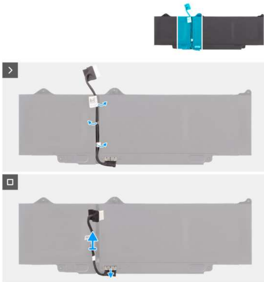
Rysunek 25. Wymontowywanie kabla baterii
