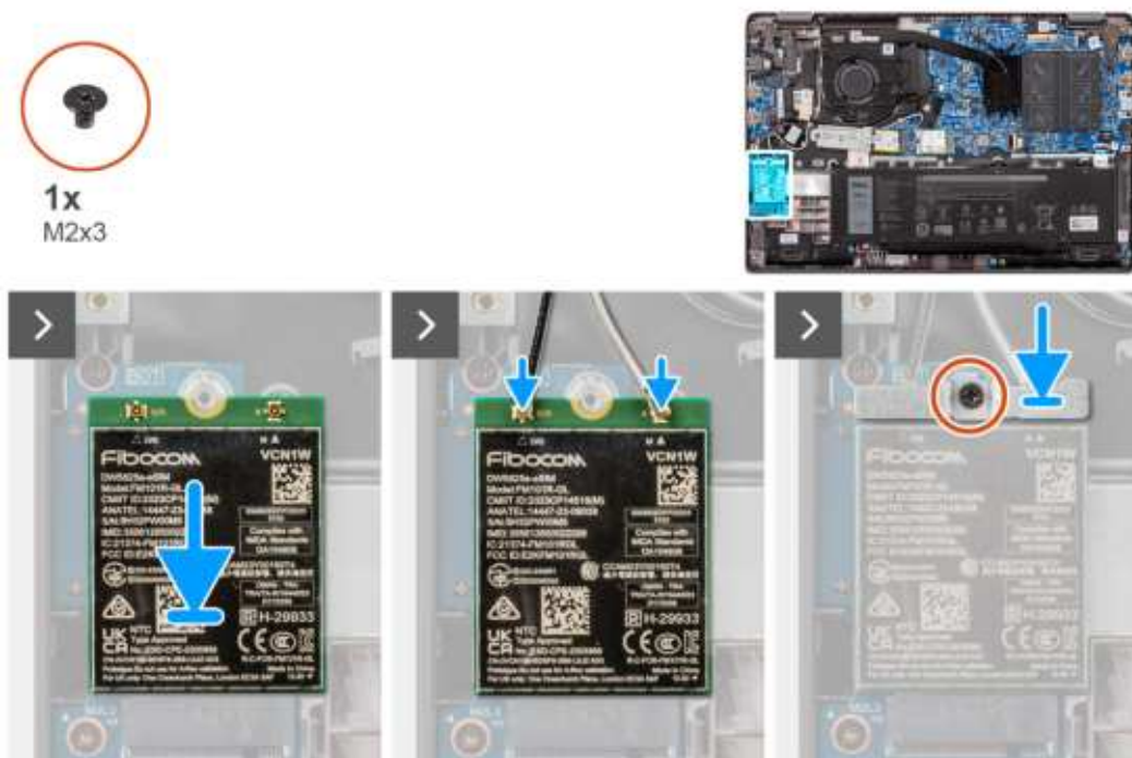
Rysunek 17. Instalowanie karty sieci WWAN
