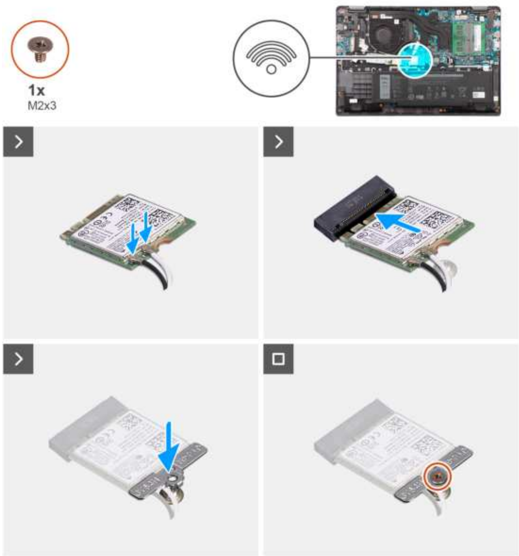
Rysunek 15. Instalowanie karty sieci bezprzewodowej
