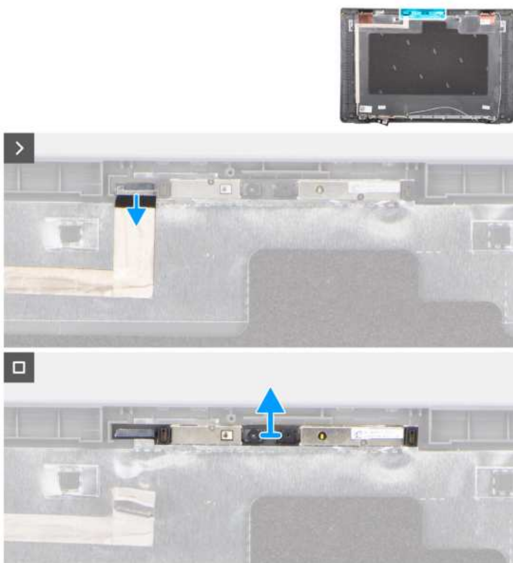
Rysunek 66. Wymontowywanie kamery
