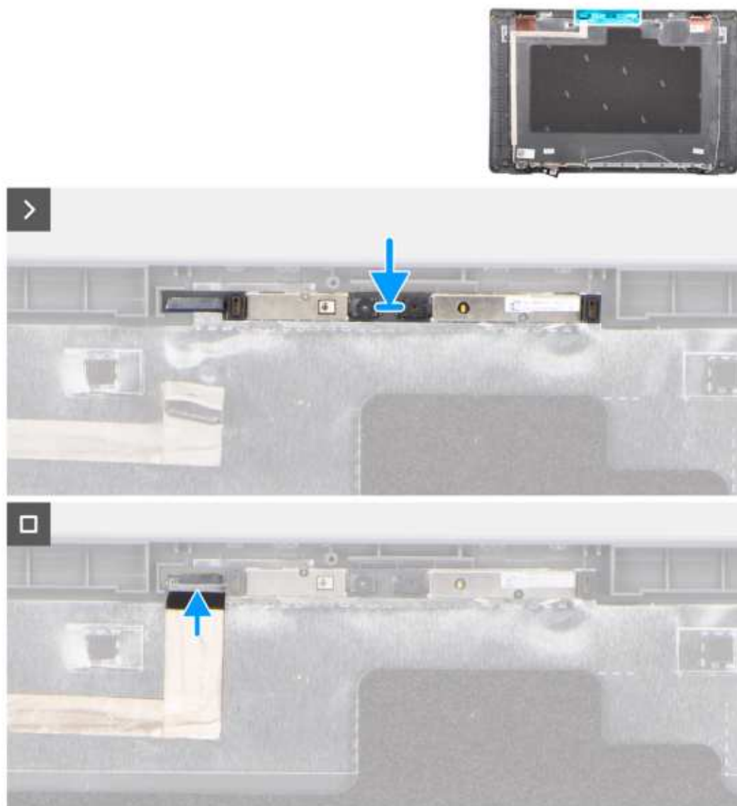
Rysunek 67. Instalowanie kamery
