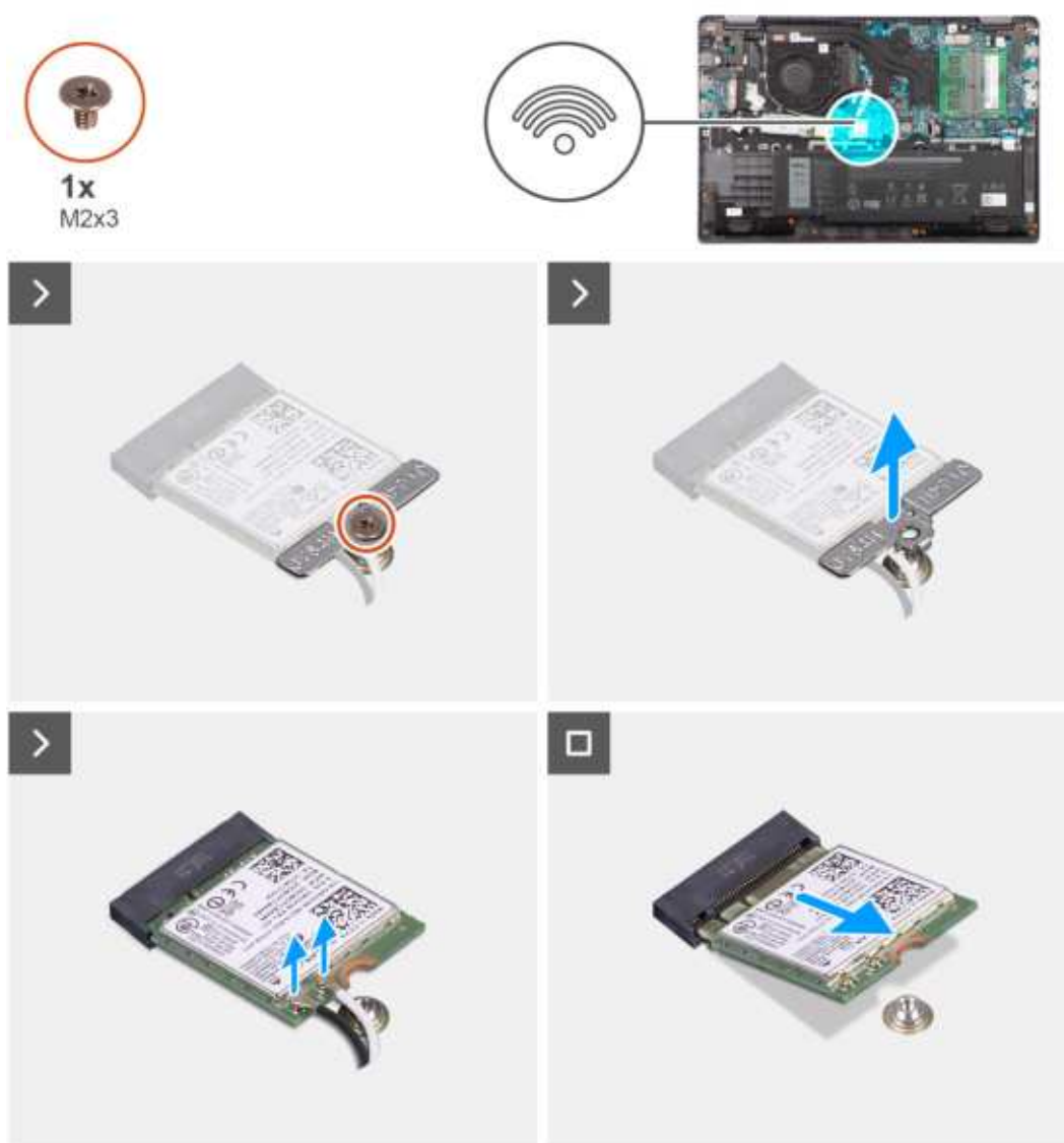
Rysunek 14. Wymontowywanie karty sieci bezprzewodowej
