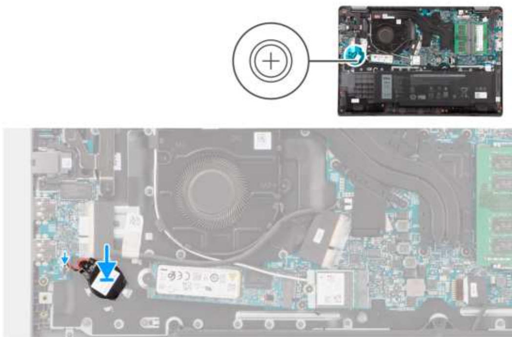
Rysunek 19. Instalowanie baterii pastylkowej
