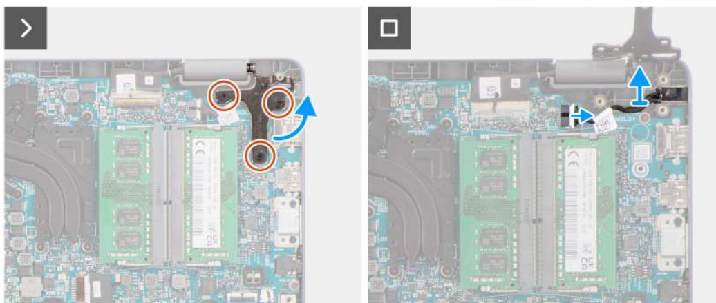
Rysunek 27. Wymontowywanie gniazda zasilacza
