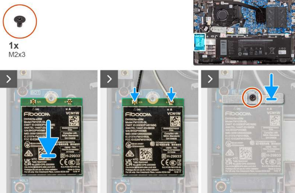
Rysunek 17. Instalowanie karty sieci WWAN
