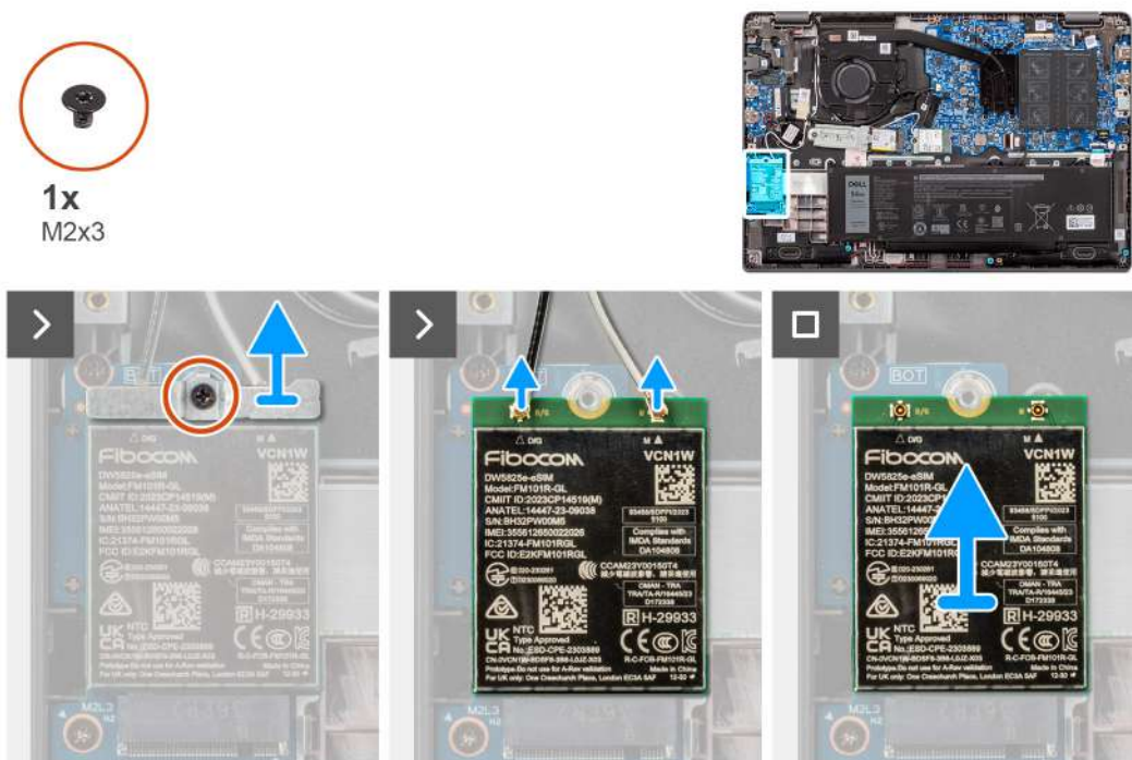
Rysunek 16. Wymontowywanie karty sieci WWAN
