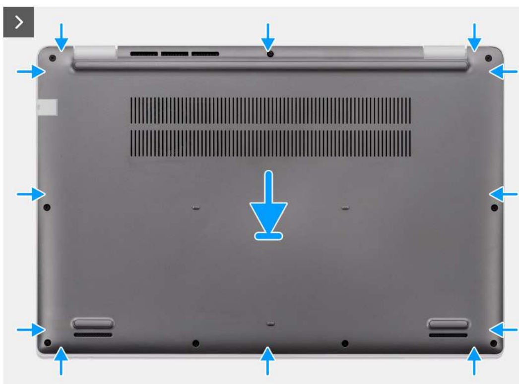
Rysunek 10. Instalowanie pokrywy dolnej
