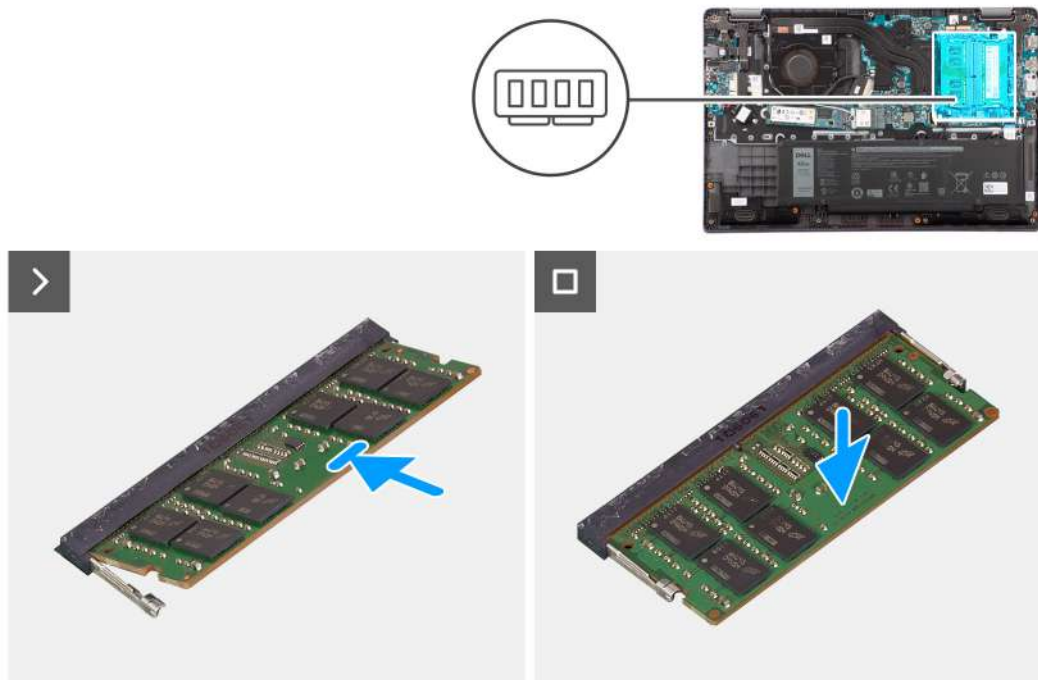
Rysunek 12. Wymontowywanie modułu pamięci
