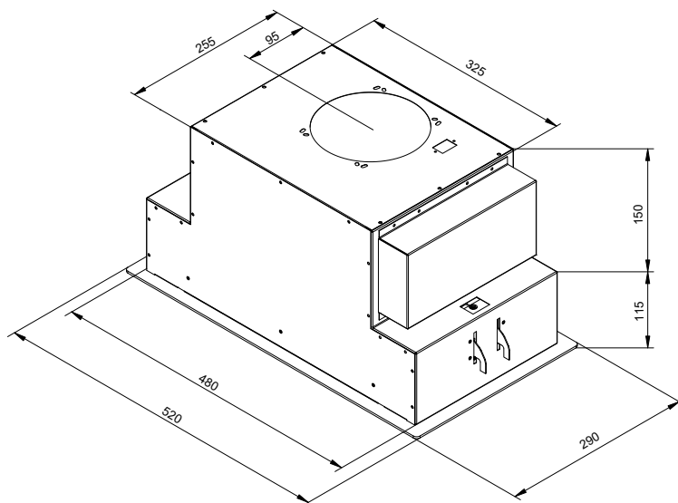
Rys.2 Rysunek gabarytowy okapu
