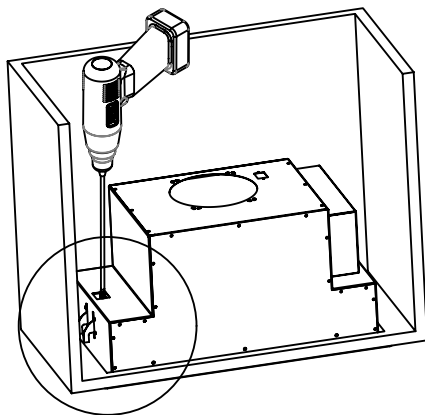
Rys. 6 Montaż korpusu okapu do szafki
