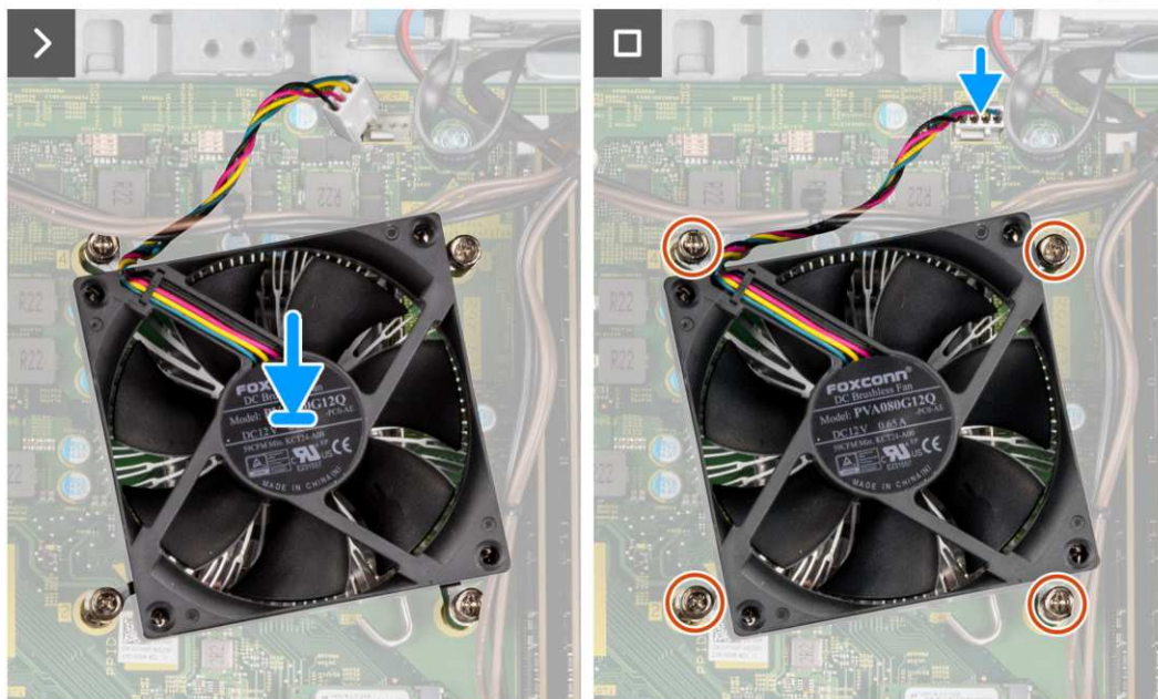
Rysunek 63. Instalowanie zestawu wentylatora i radiatora procesora
