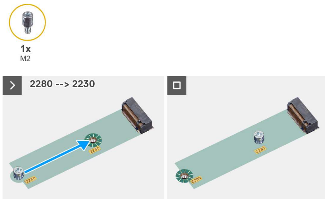
Rysunek 20. Instalowanie dysku SSD M.2 2230
