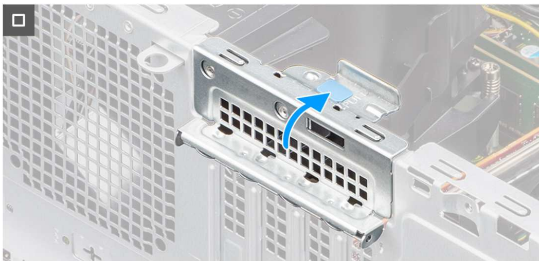
Rysunek 73. Wymontowywanie opcjonalnego modułu złącza PS2/szeregowego
