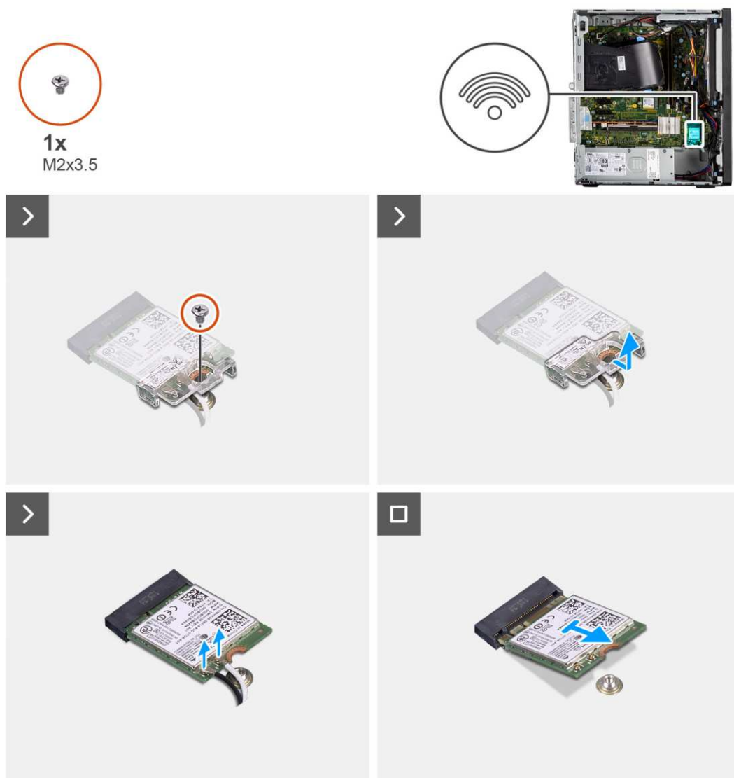
Rysunek 31. Wymontowywanie karty sieci bezprzewodowej
