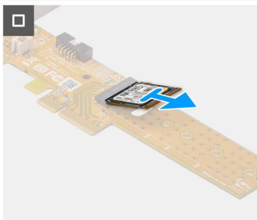
Rysunek 26. Wymontowywanie dysku SSD M.2 2230 na karcie Dell Ultra Speed Drive trzeciej generacji
