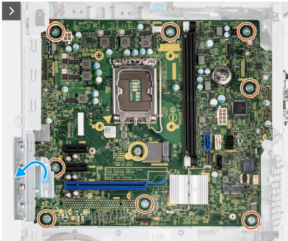
Rysunek 85. Wymontowywanie płyty głównej
