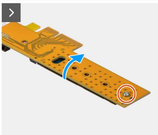
Rysunek 29. Instalowanie dysku SSD M.2 2280 na karcie Dell Ultra Speed Drive trzeciej generacji
