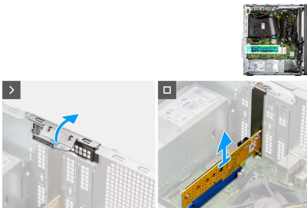
Rysunek 25. Wymontowywanie karty Dell Ultra Speed Drive trzeciej generacji
