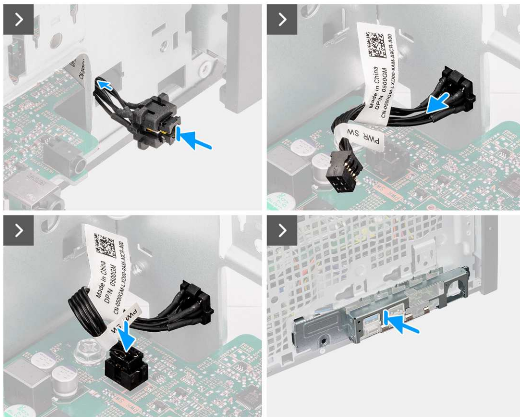
Rysunek 50. Instalowanie przycisku zasilania
