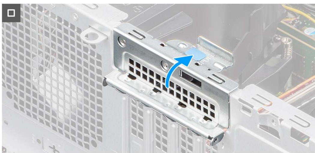
Rysunek 75. Instalowanie opcjonalnego modułu złącza PS2/szeregowego
