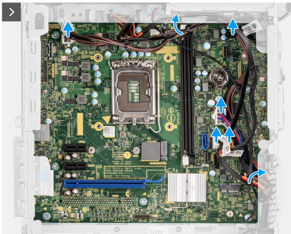
Rysunek 84. Wymontowywanie płyty głównej
