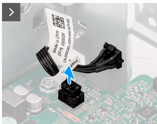
Rysunek 49. Wymontowywanie przycisku zasilania
