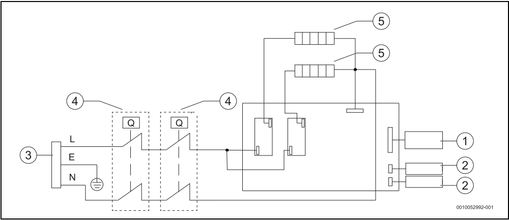
Rys. 17 Schemat połączeń
