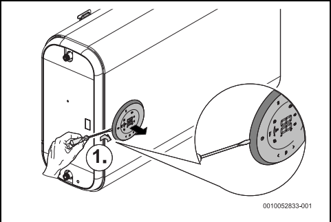
Rys. 12 Odłączanie wyświetlacza
