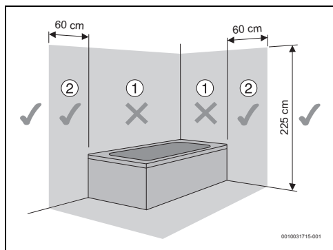
Rys. 7 Strefa ochronna
