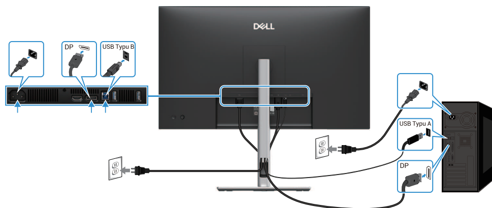
Rysunek 28. Podłączanie kabla DisplayPort i USB
