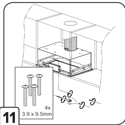
Sposób montażu do szafki 60cm
