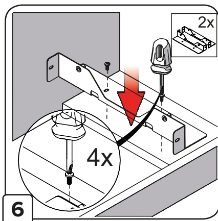
Sposób montażu do szafki 80/90cm
